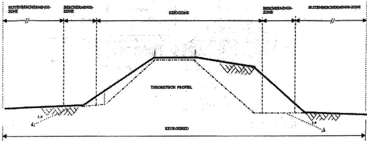
ZIJAAZICHT THEORETISCH PROFIEL VAN EEN WATERKERING
