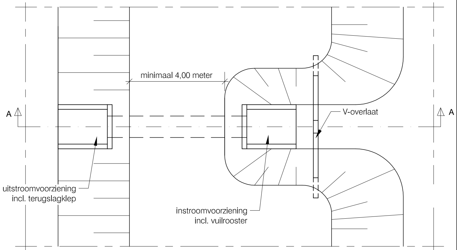
Bovenaanzicht
