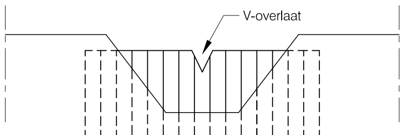
Vooraanzicht
