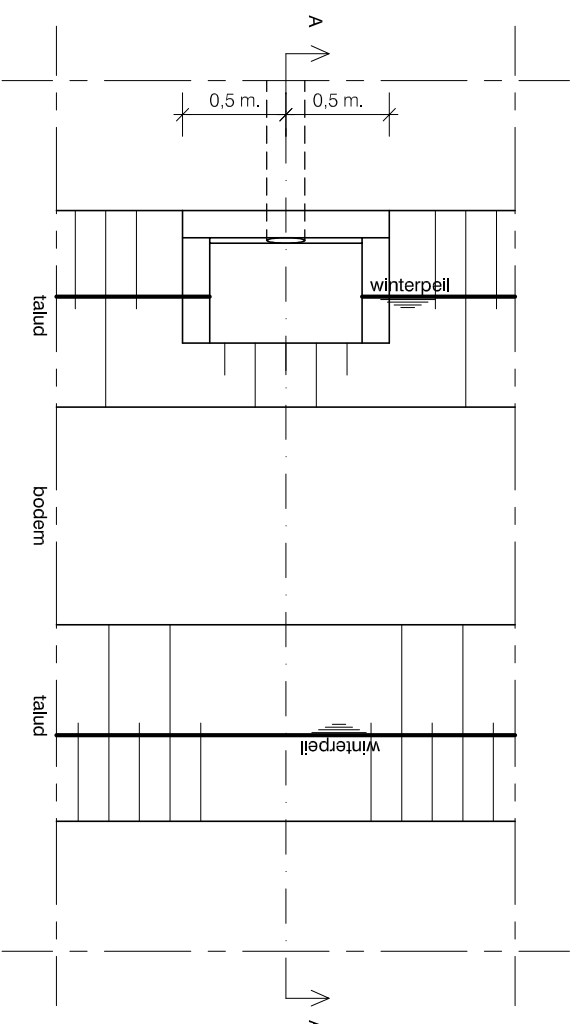
Bovenaanzicht
