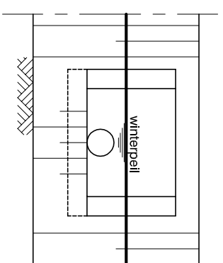
Vooranzicht
