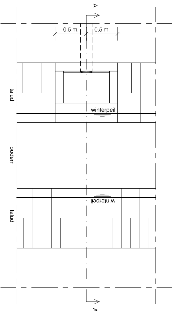
Bovenaanzicht
