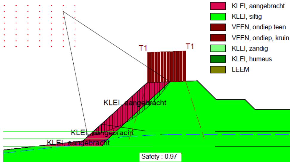
Figuur 3-2: Doorsnede DP4 van Fort Henricus. Aan de buitenzijde van het talud is 1,5 m klei aangebracht.
