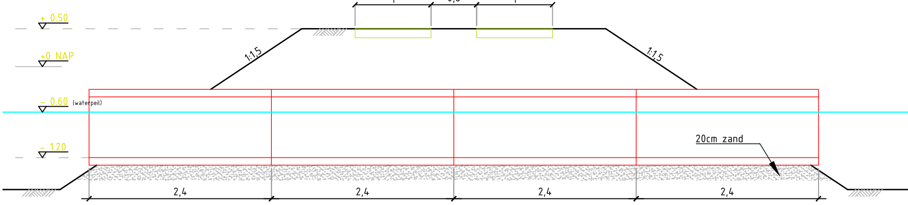
Dwarsdoorsnede AA' - schaal 1:50
