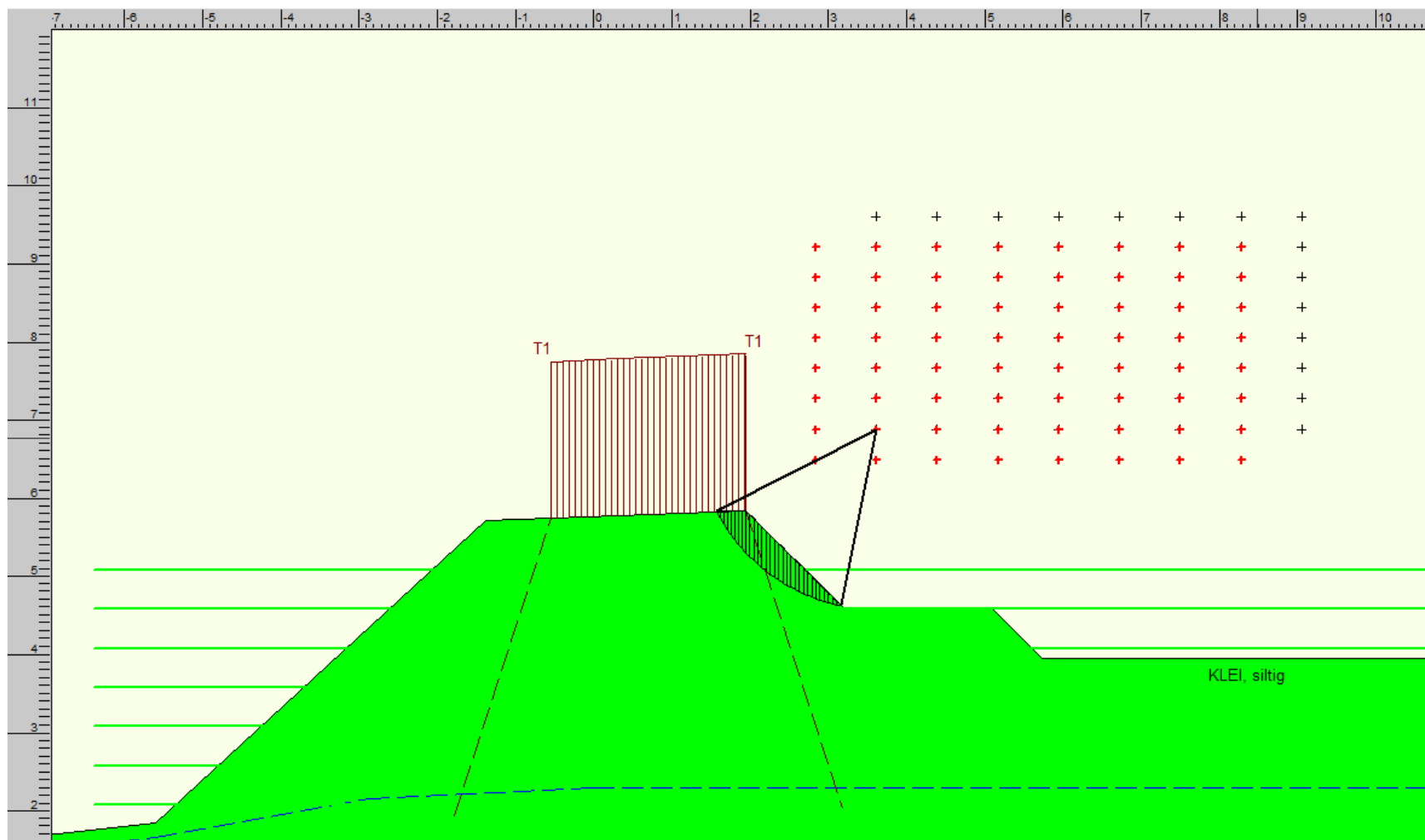
Figuur B2: Berekende maatgevende glijcirkel binnenwaarts bij fort Henricus met methode Bishop. Stabiliteitsfactor 1,12 (eis 1,00).
