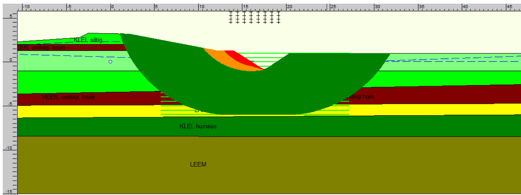
Figuur B7: Berekenende glijcirkel bij boezemkade voor de huidige situatie met methode Bishop. Stabiliteitsfactor 0,81 (eis 1,08).
