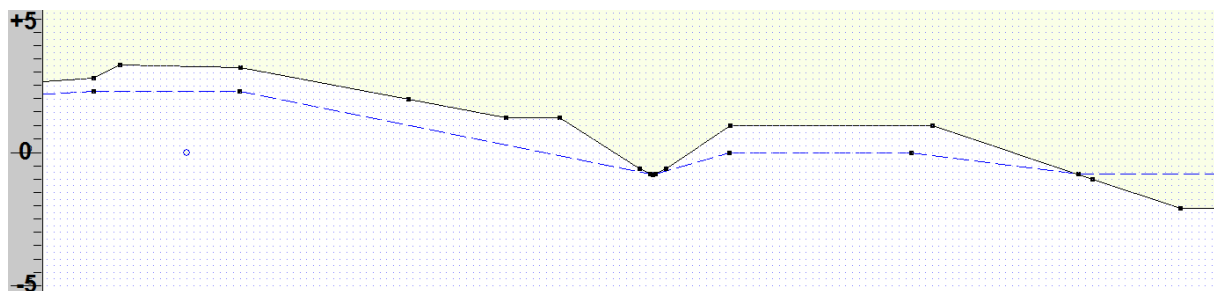
Figuur 2-2: Grondwaterstandsverloop (blauw lijn) bij boezemkade in meters boven NAP
