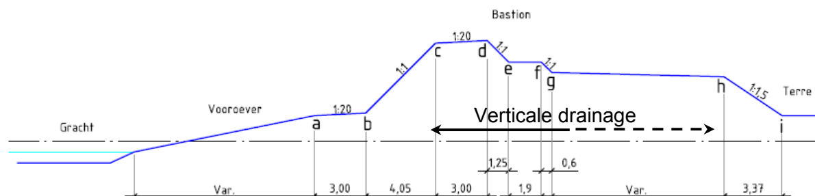
Figuur 3-4: Principeddoorsnede taluds, en ligging verticale drainage (GKB, feb 2016)
