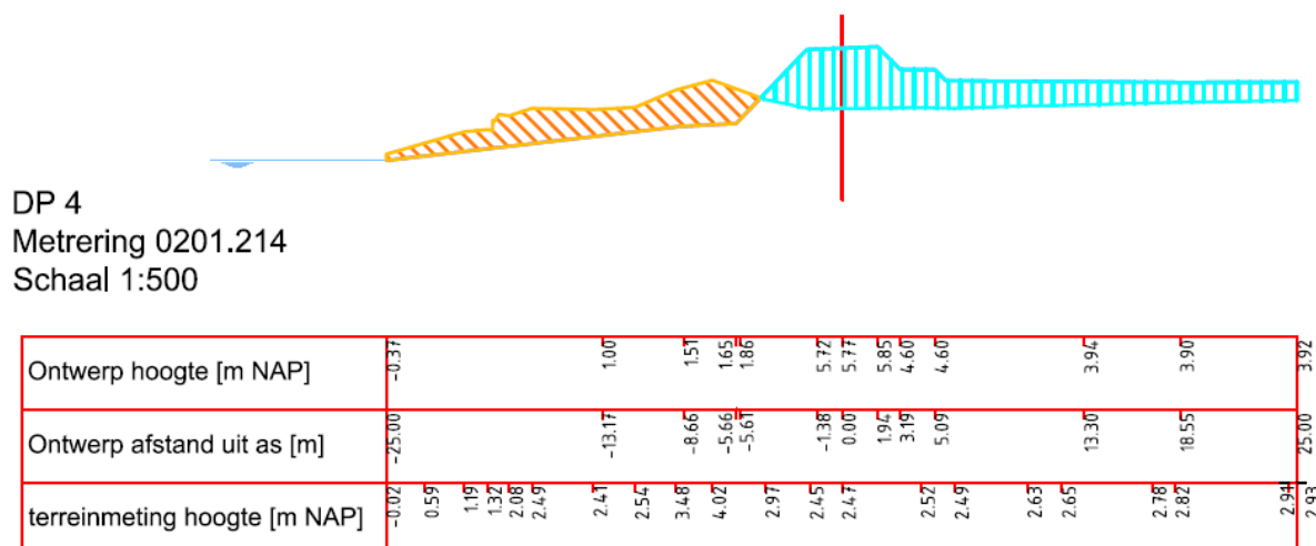
Figuur 3-1: Doorsnede DP4 van Fort Henricus. De maximale ophoging bedraagt ca. 3,3 m.
