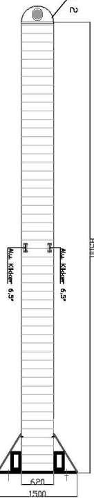
BA Vingerpier VP400-620-700HD01 Aantal 02 stuks boxnr. 135 t/m 138
