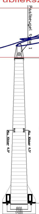
BA Vingerpier VP400-400/800-700HD01 Aantal 12 stuks box nr 80t/m 102
