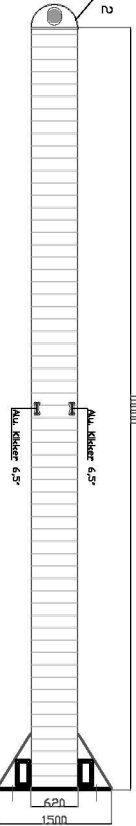
BA Vingerpier VP400-620-700HD01 Aantal 06 stuks boxnr 16 t/m 21 en 26 t/m 31
