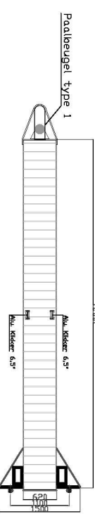
BA Vingerpier VP400-620-700HD01 Aantal 04 stuks boxnr. 103t/m 111
