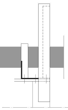
Z.A RVS beugel t.p.v vaste vingerpier bev. aan kade
