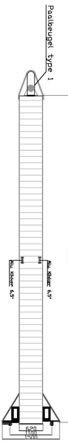
BA Vingerpier VP400-620-700HD01 Aantal 06 stuks boxnr. 1t/m 7 en 139t/m 143
