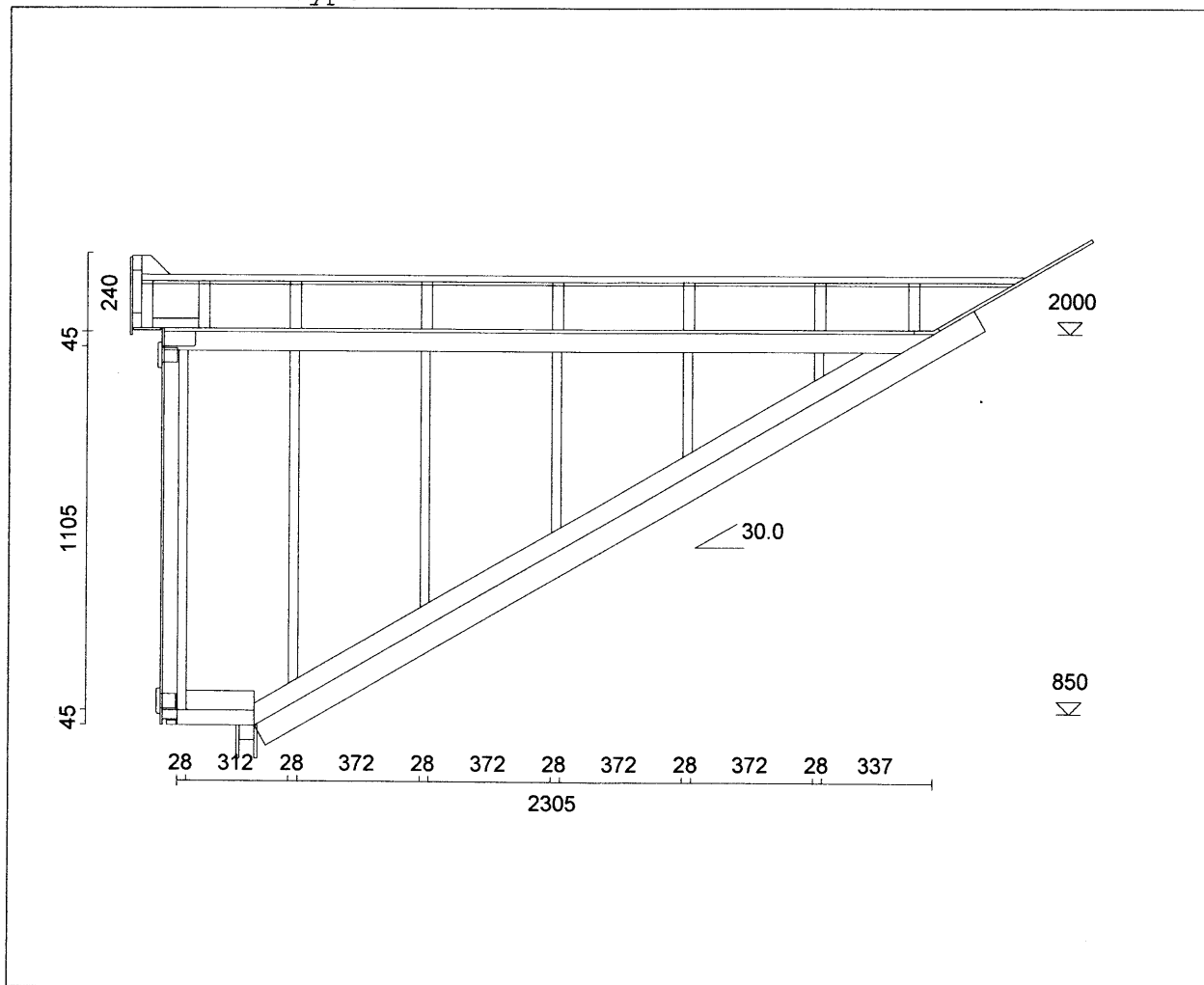
Dwarsdoorsnede type E
