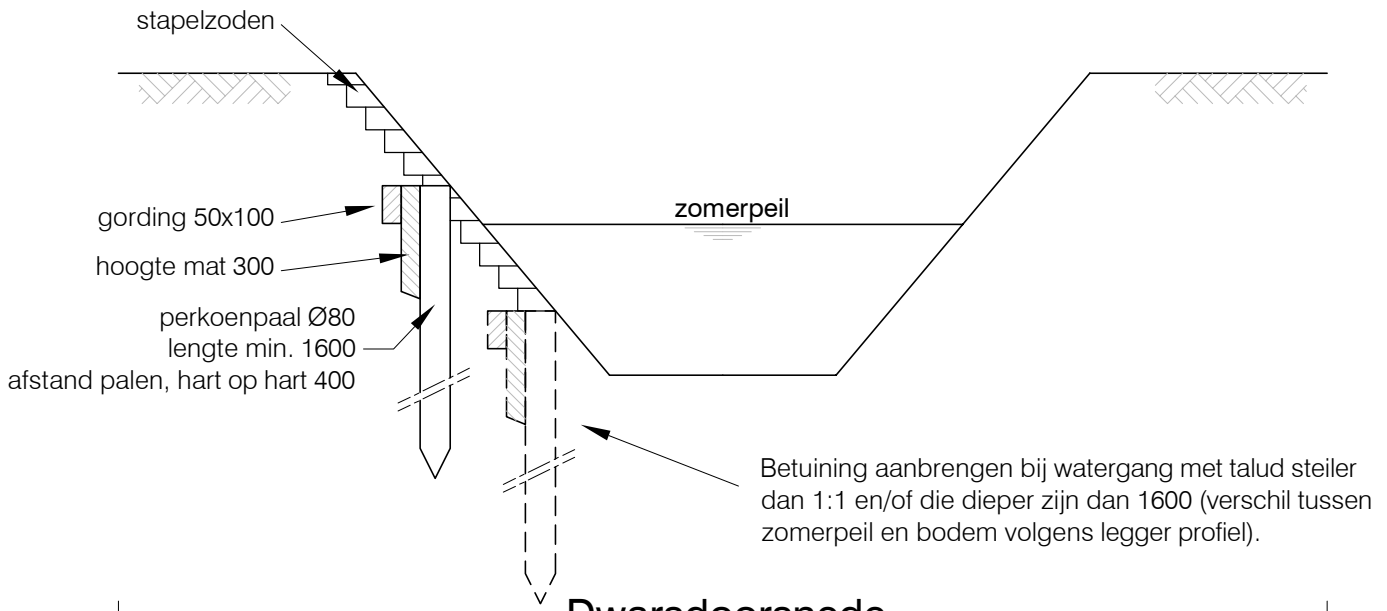
Dwarsdoorsnede
