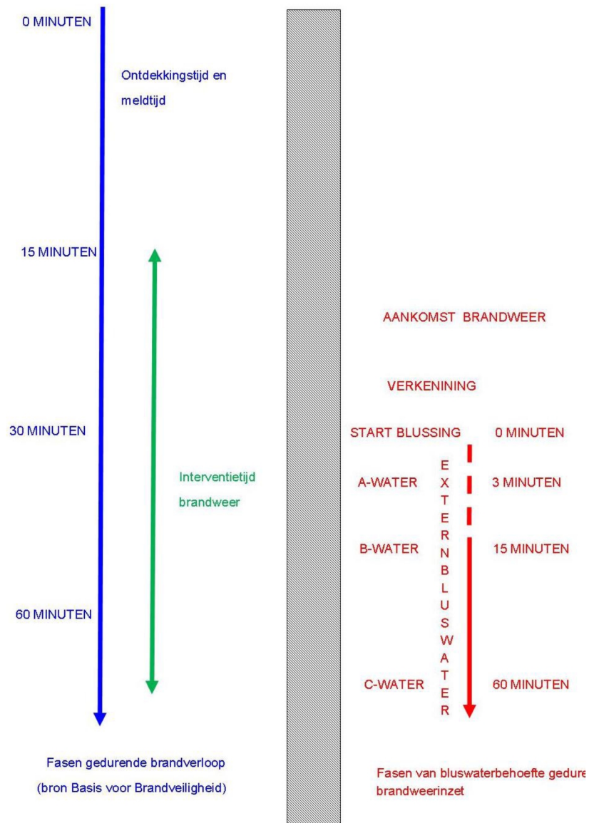
Figuur 12 Schematische weergave van bluswaterbehoefte gerelateerd aan fasen van brandverloop (tijdbalken zijn niet op schaal).
