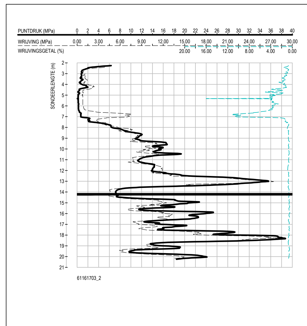
SONDERING 61161703_2 SCHAAL 1:200
