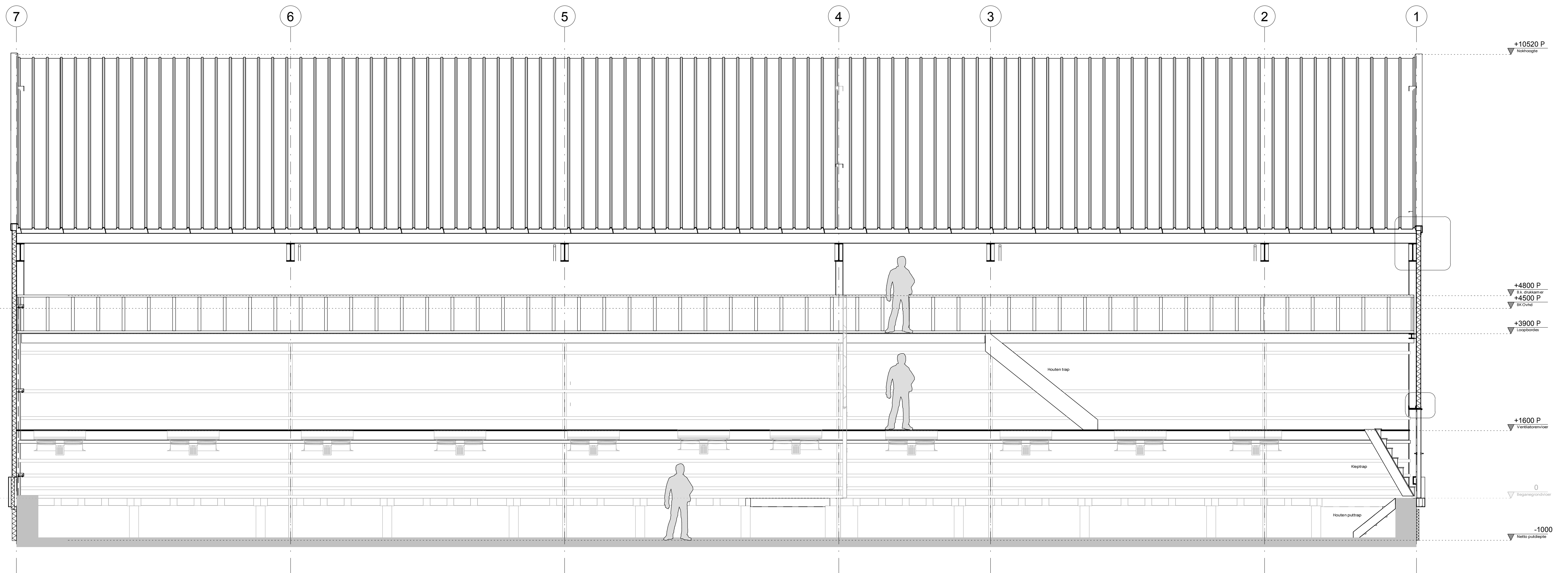
DOORSNEDE B-B 1:50
