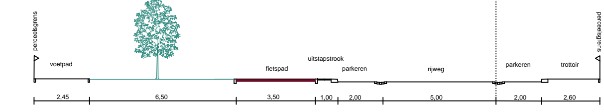
nieuw dwarsprofiel B - B1
