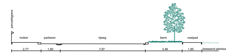
bestaand dwarsprofiel A - A1
