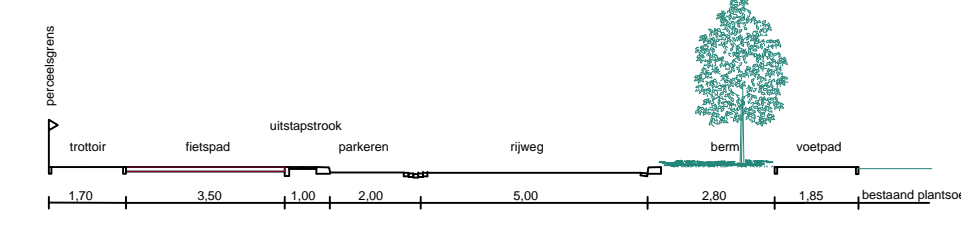
nieuw dwarsprofiel A - A1
