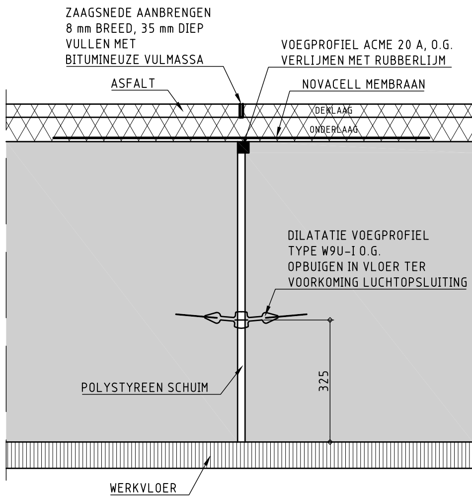
BUITENZIJDE WAND VLOER
