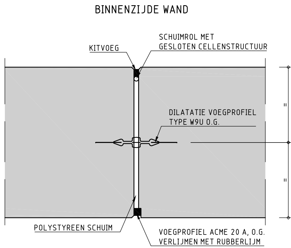
BINNENZIJDE WAND WAND
