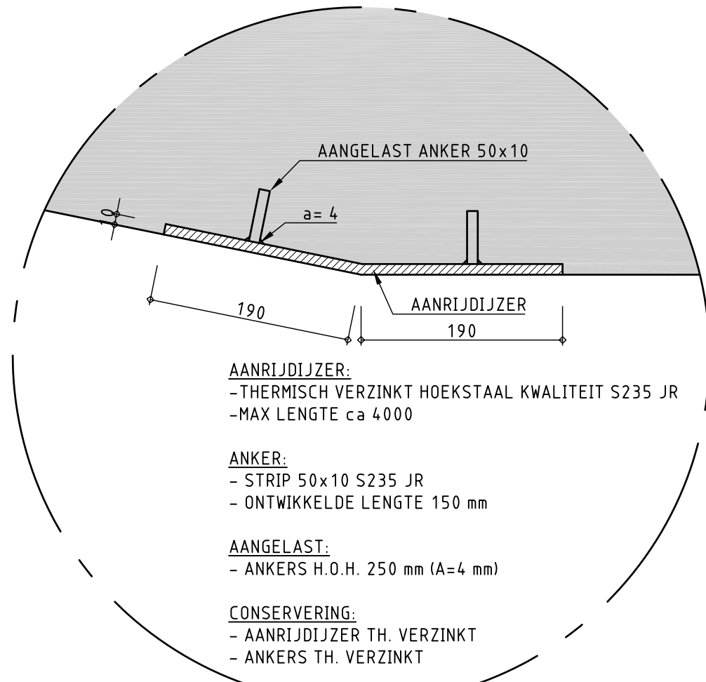
DETAIL AANRIJDIJZER SCHAAL 1:5
