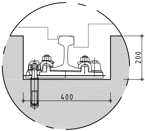
DETAIL INKASSING DEK SCHAAL 1:10
