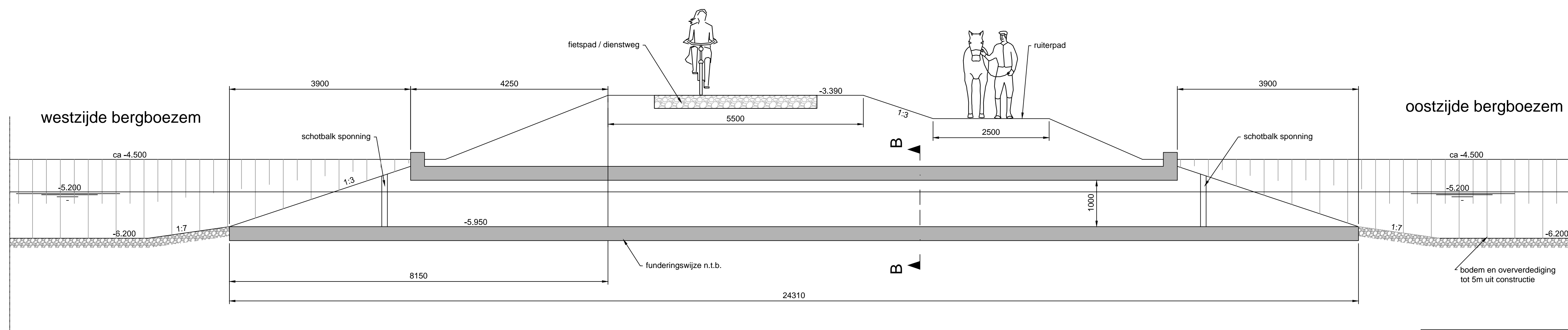
Langsdoorsnede A-A
