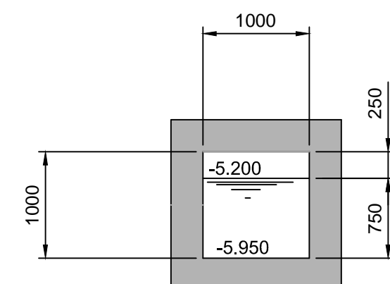
Doorsnede B-B
