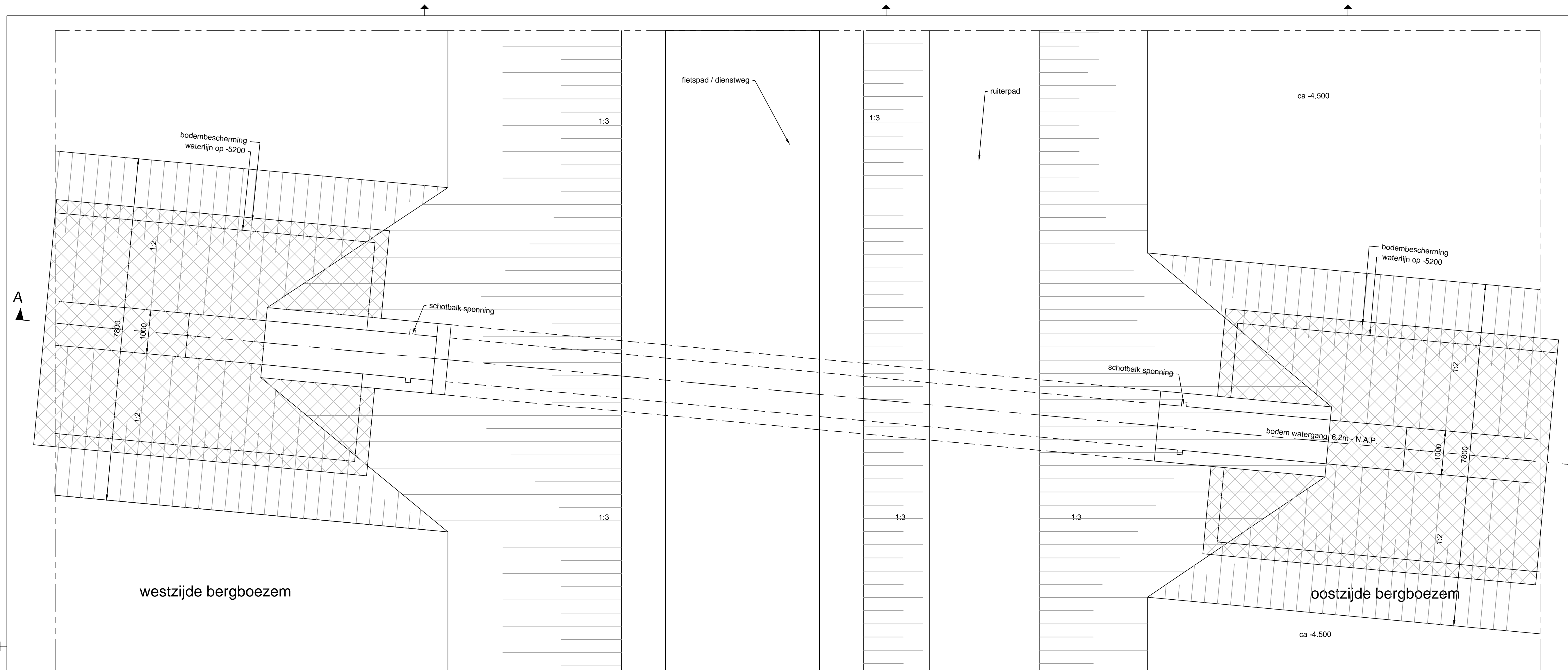
Bovenaanzicht
