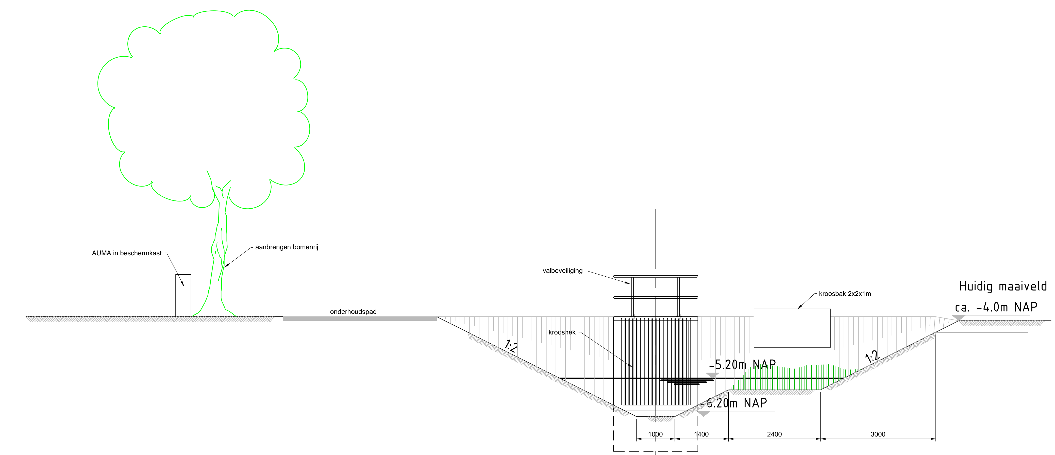
Vooraanzicht B-B
