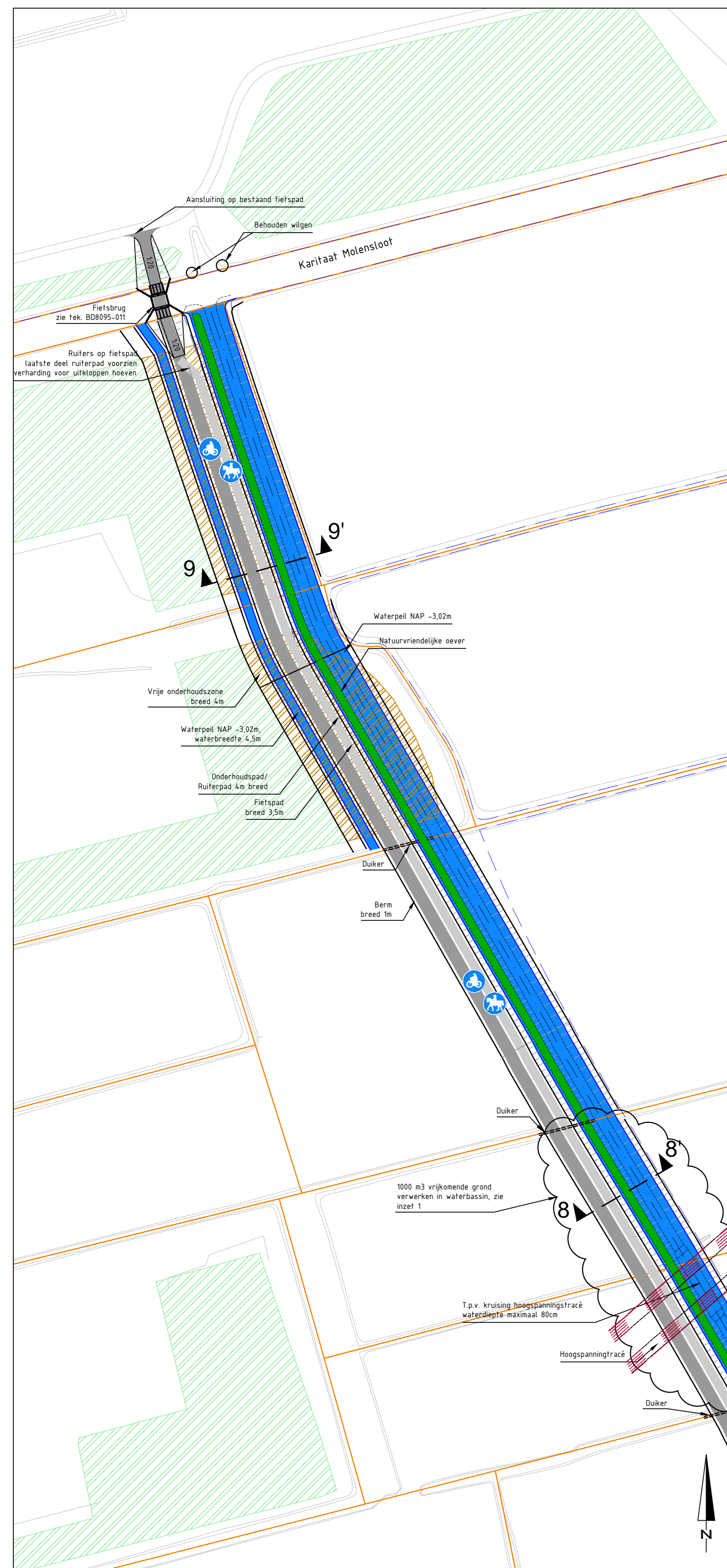
Situatie 2: Noord-zuid verbinding Schaal: 1:1000
