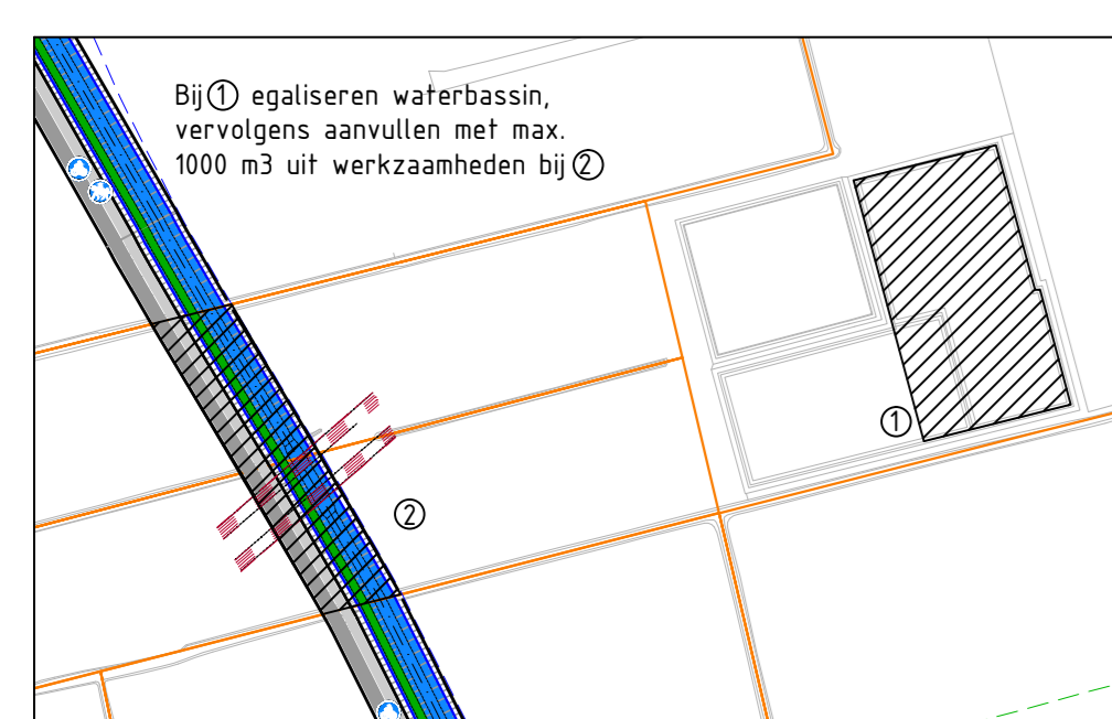
Situatie 3: Werkzaamheden perceel Van Boxtel Schaal: 1:2500
