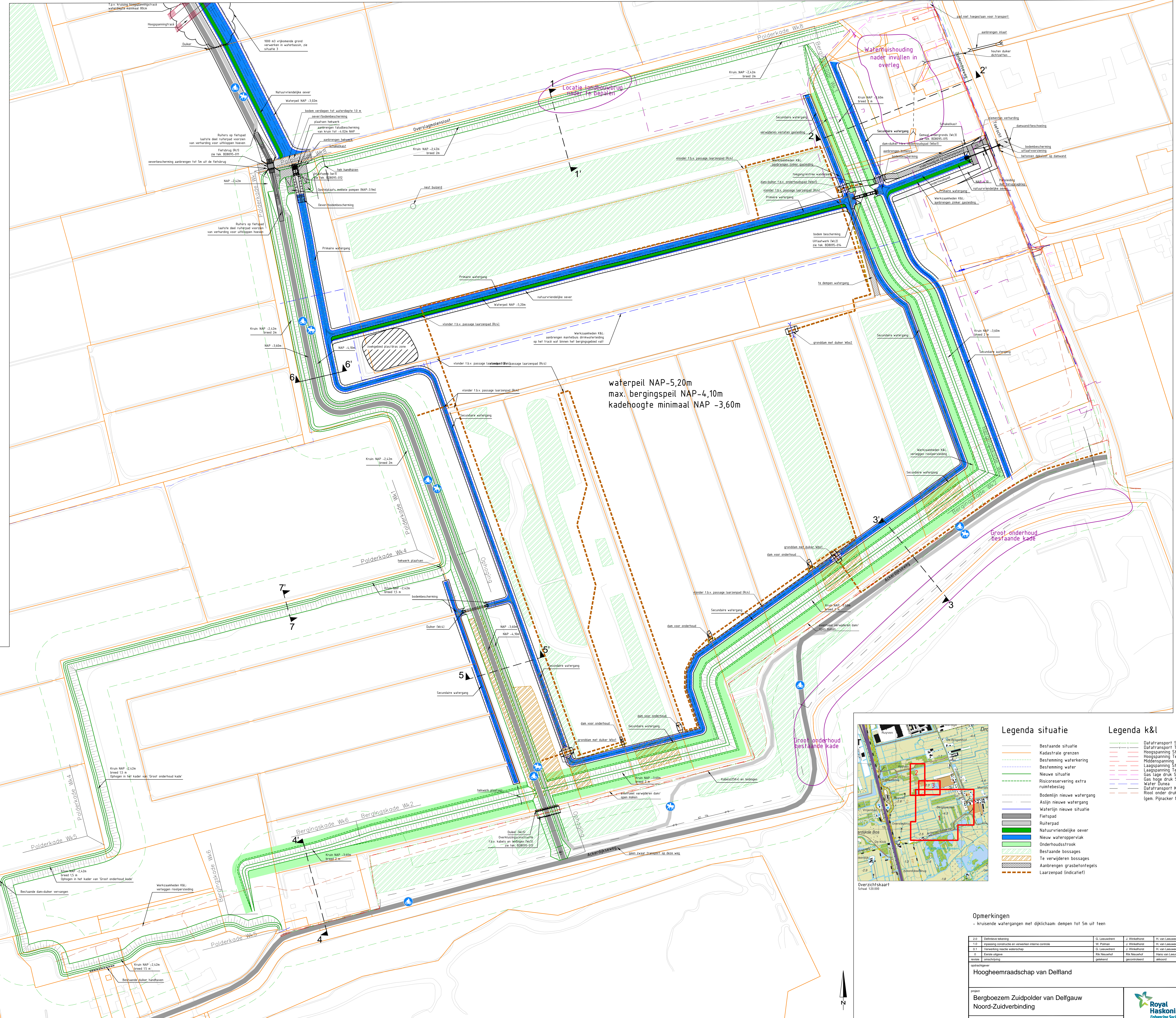
Situatie 1: Bergboezem Zuidpolder van Delfgauw Schaal: 1:1000
