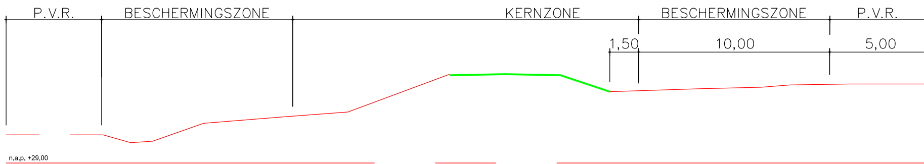
DWARSPROFIEL 50.510.13 SCHAAL 1:200
