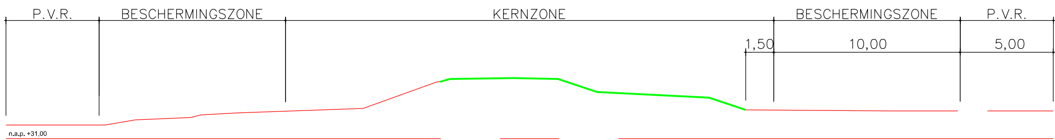
DWARSPROFIEL 50.510.11 SCHAAL 1:200
