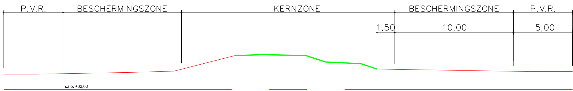
DWARSPROFIEL 50.510.09 SCHAAL 1:200
