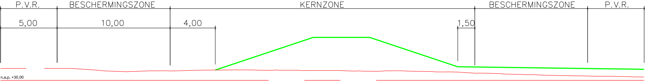
DWARSPROFIEL 50.510.N01 SCHAAL 1:200
