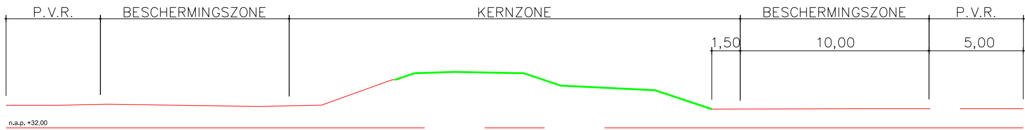
DWARSPROFIEL 50.510.10 SCHAAL 1:200
