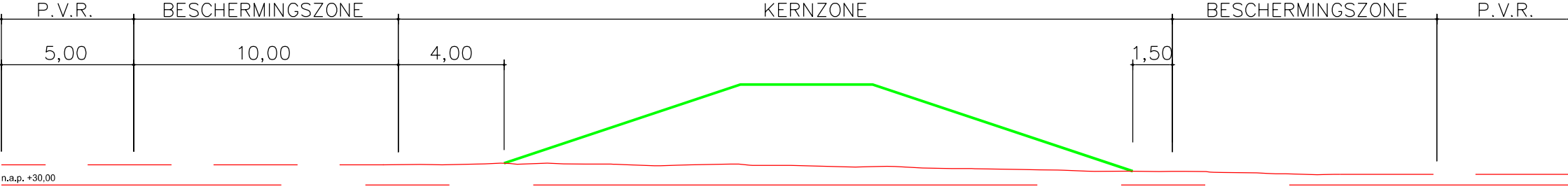
DWARSPROFIEL 50.510.N02 SCHAAL 1:200
