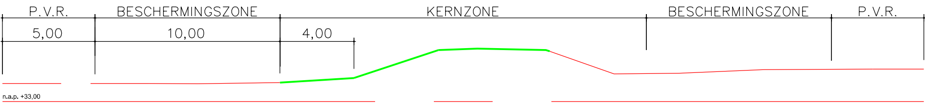
DWARSPROFIEL 50.510.01 SCHAAL 1:200
