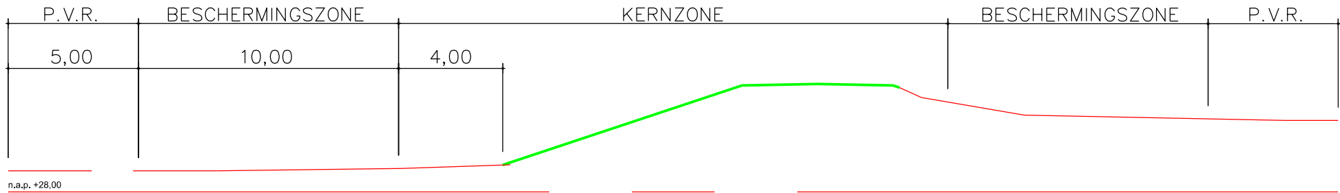
DWARSPROFIEL 50.530.16-1 SCHAAL 1:200
