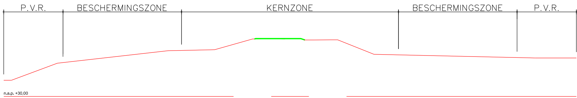
DWARSPROFIEL 50.510.08 SCHAAL 1:200
