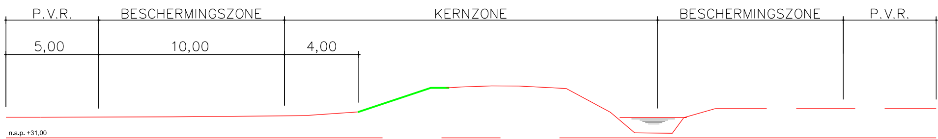
DWARSPROFIEL 50.510.12 SCHAAL 1:200
