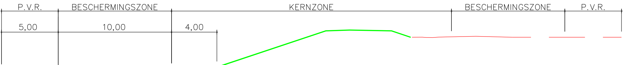
DWARSPROFIEL 50.510.06 SCHAAL 1:200
