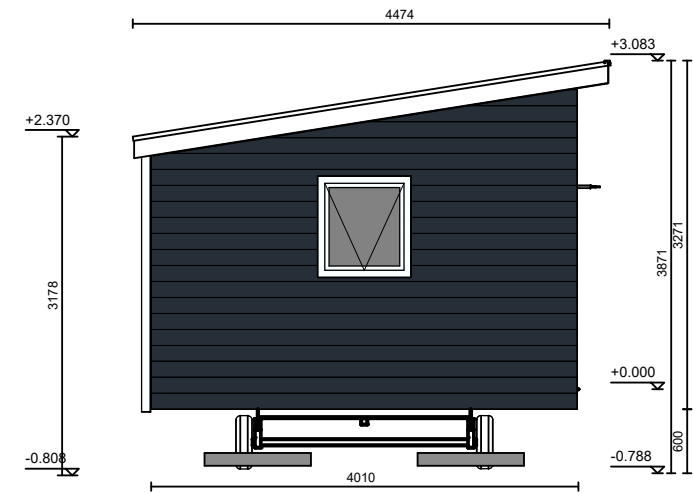
Linkeraanzicht
