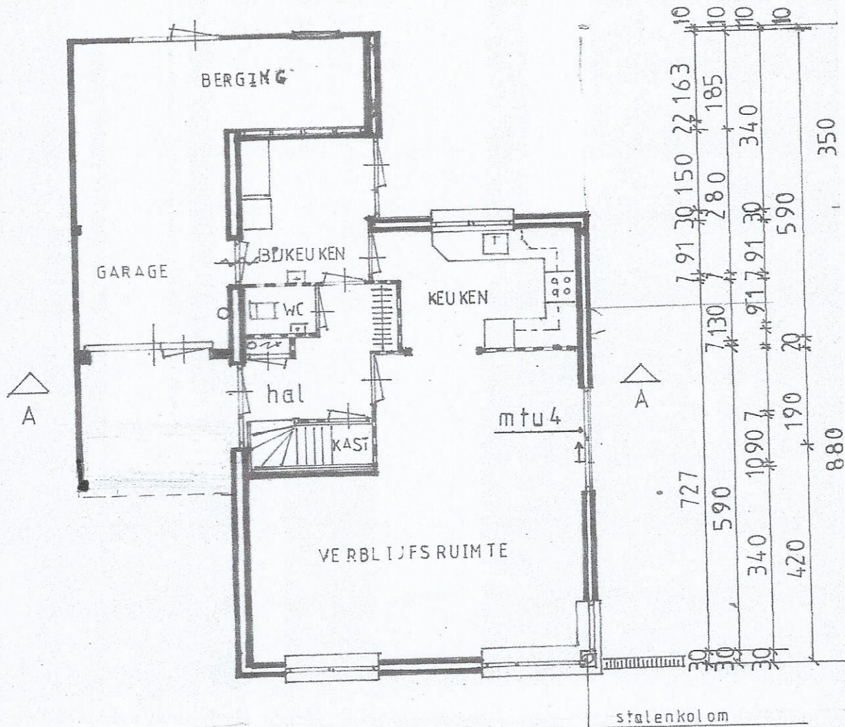
BEGANE GROND
