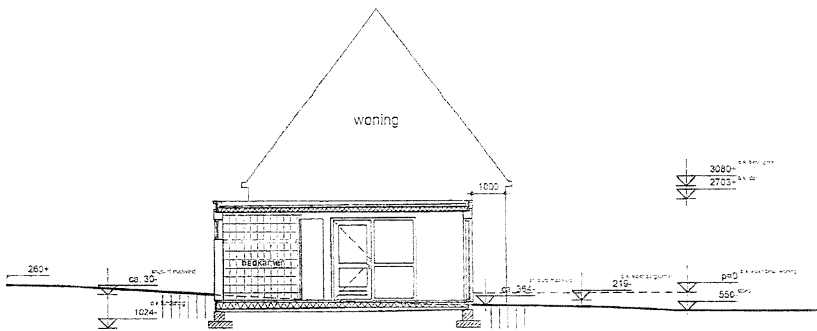
doorsnede A-A
