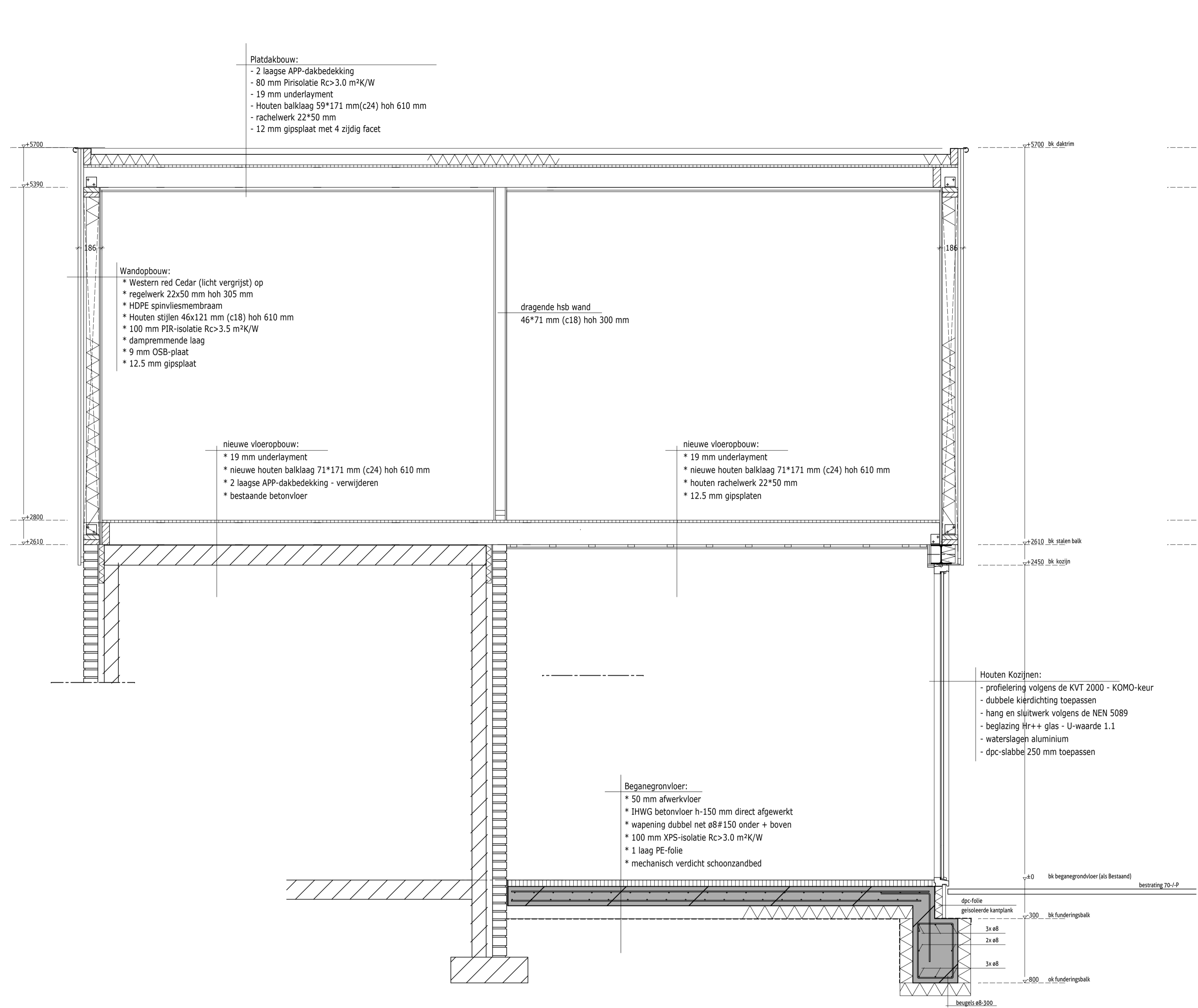
Doorsnede A-A
