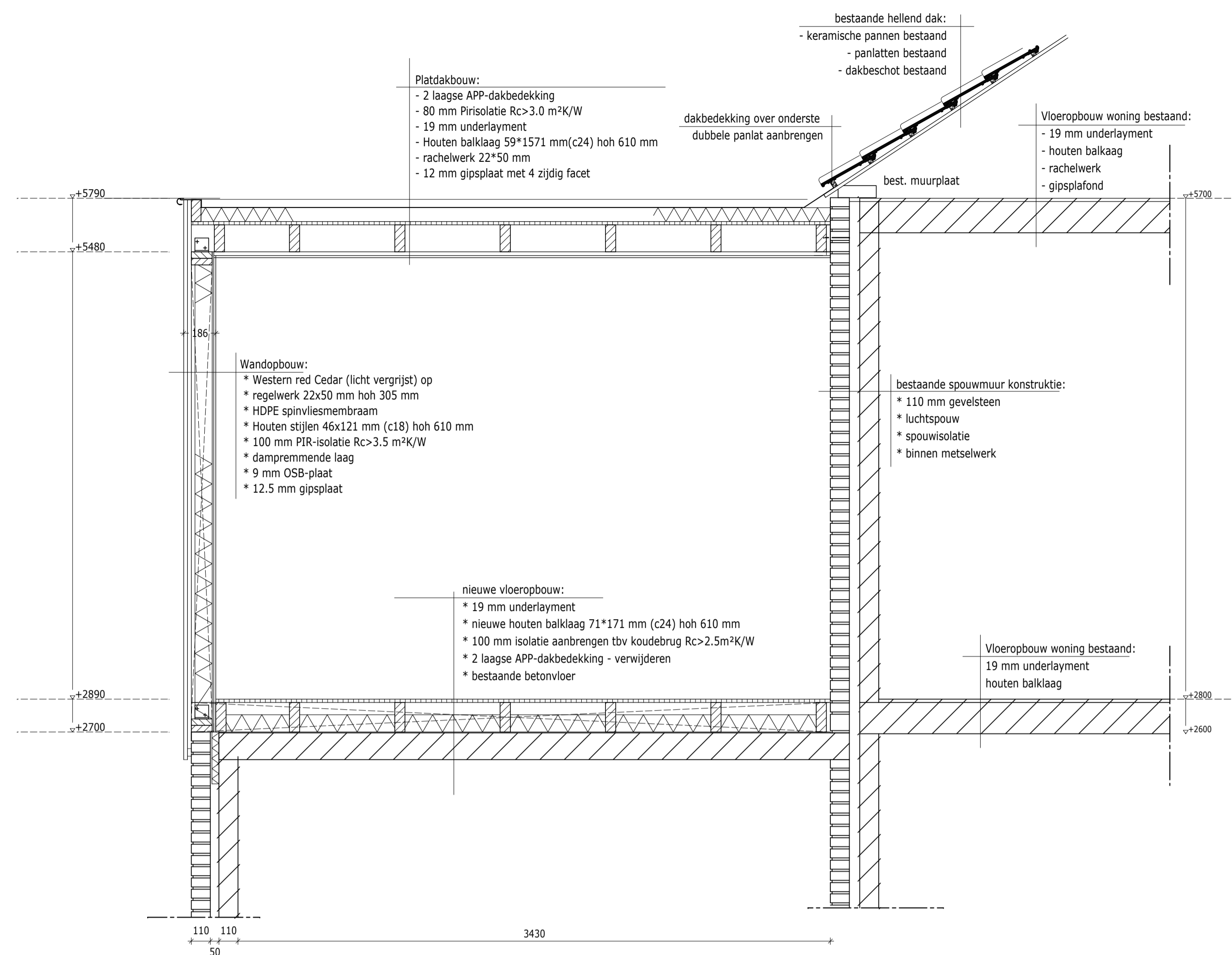
Doorsnede B-B
