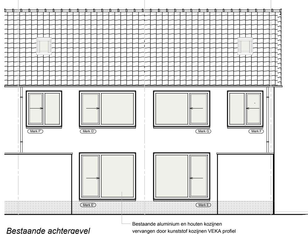
Bestaande achtergevel
