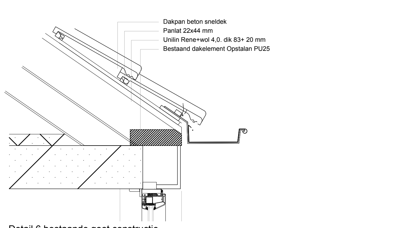
Detail 6 bestaande goot constructie
