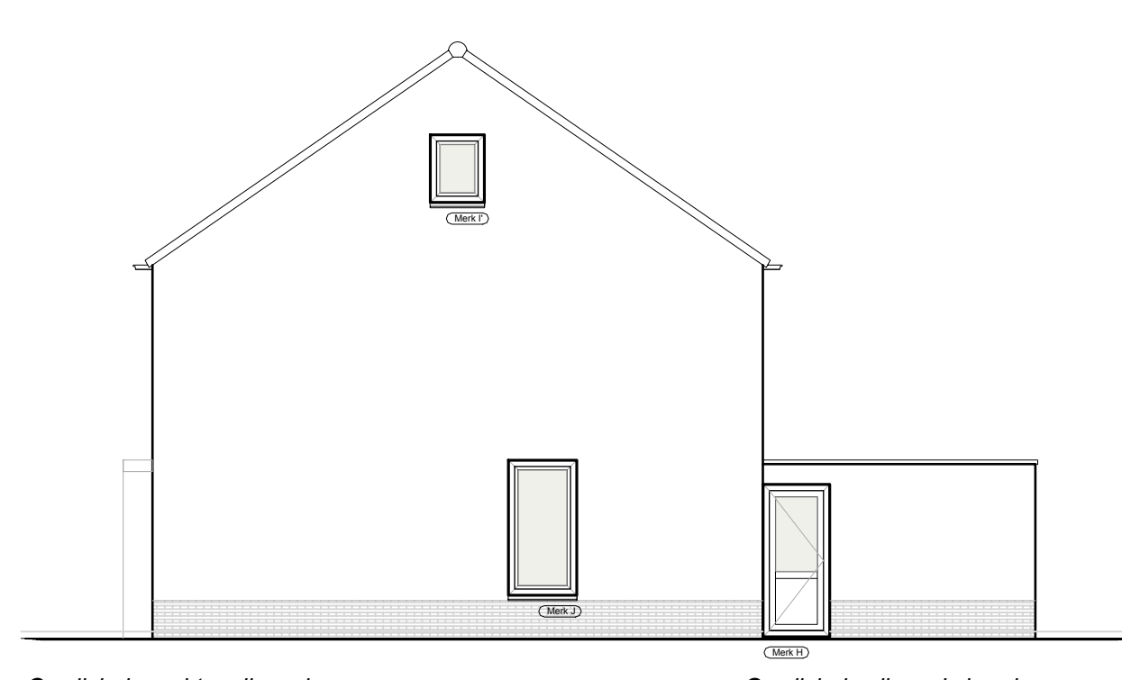
Gewijzigde rechter zijgevel
