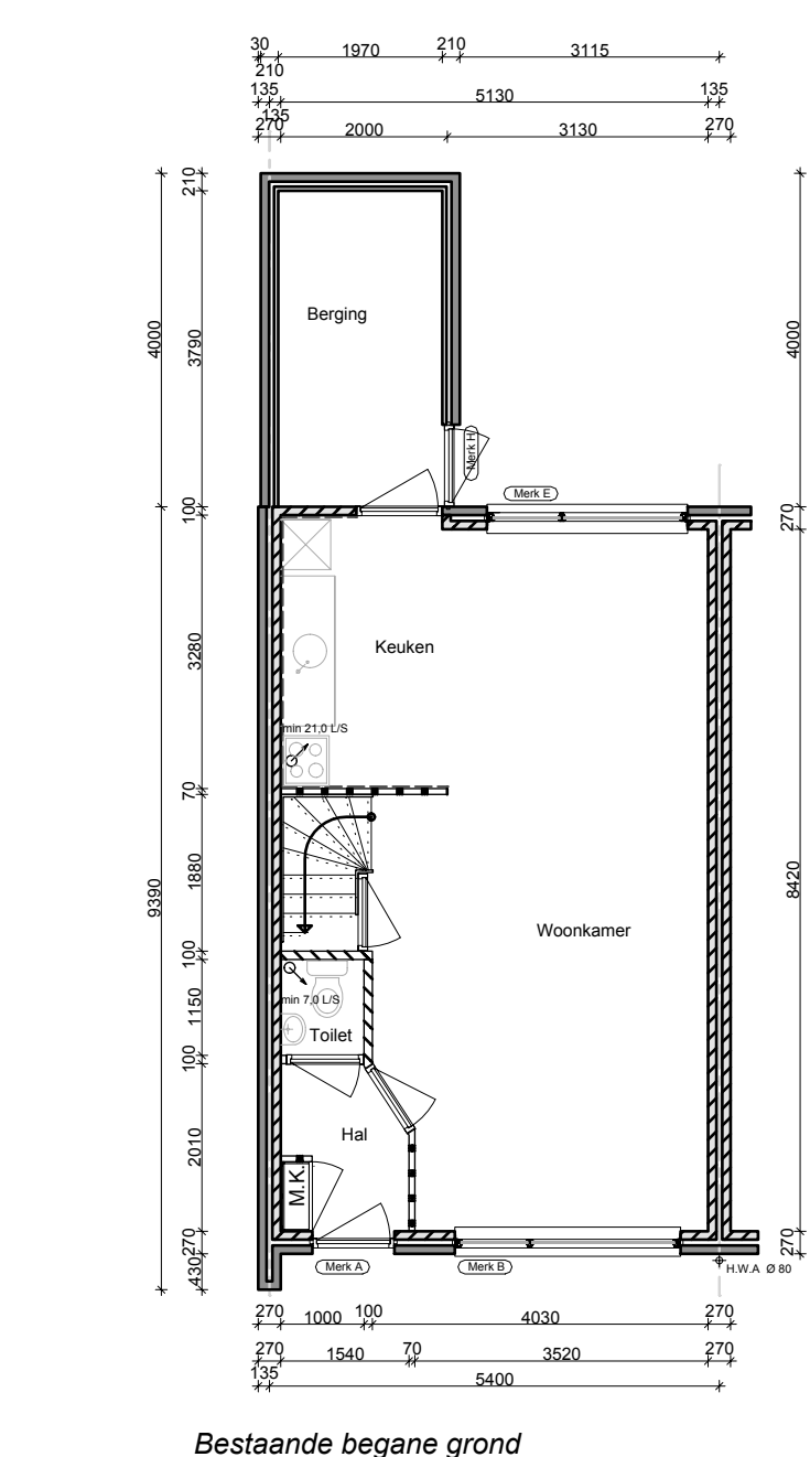
Bestaande begane grond
