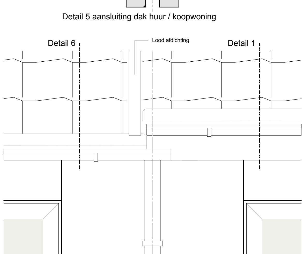
Detail 5 aansluiting dak huur / koopwoning
