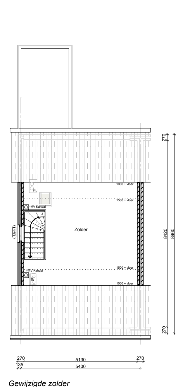
Gewijzigde zolder
