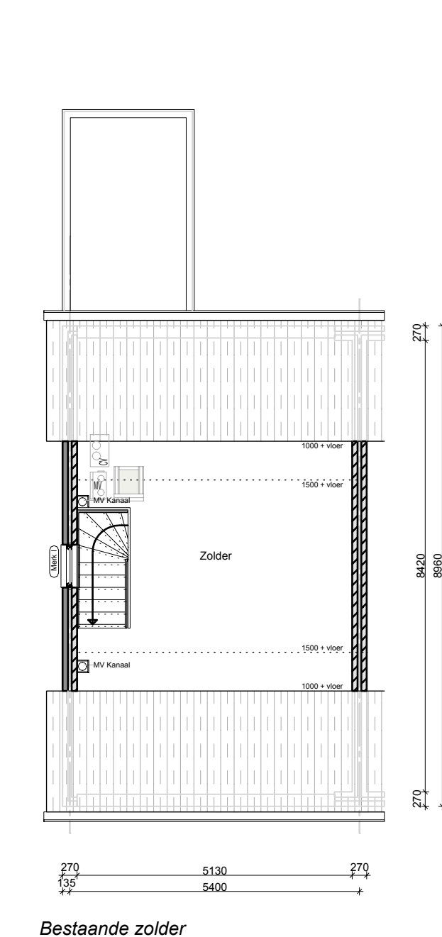
Bestaande zolder
