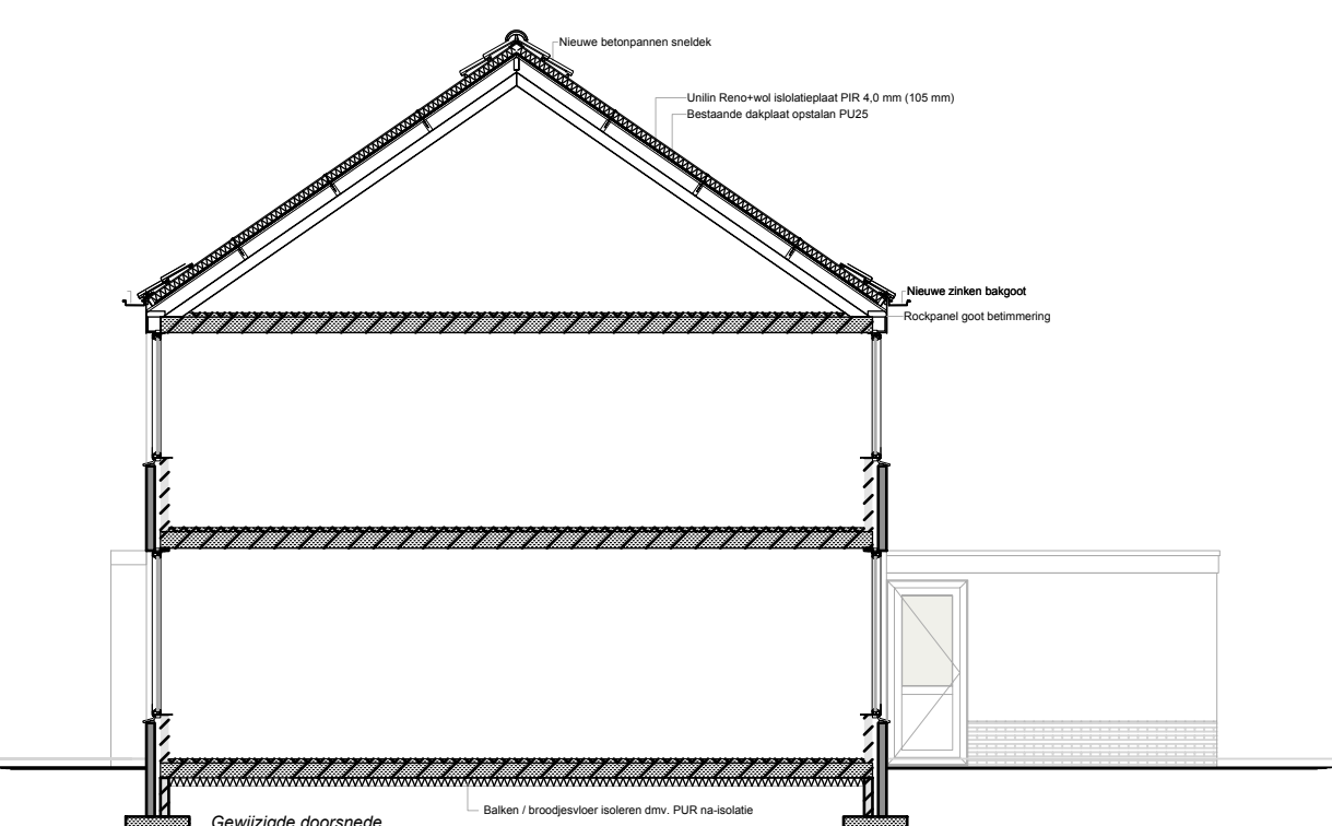
Gewijzigde deorside
