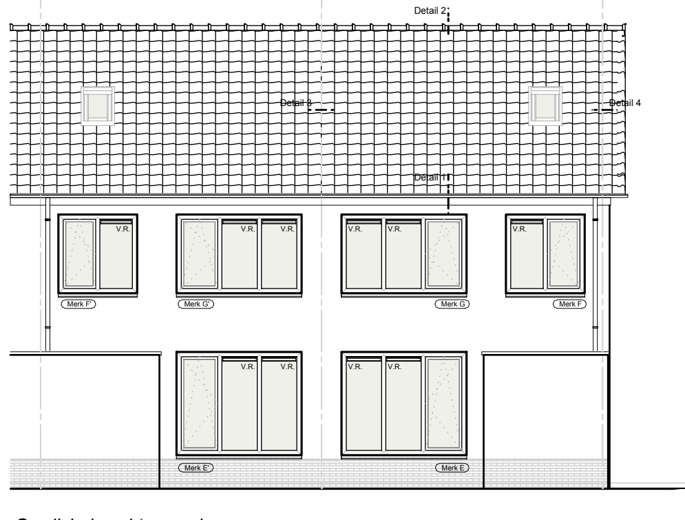
Gewijzigde achtergevel
