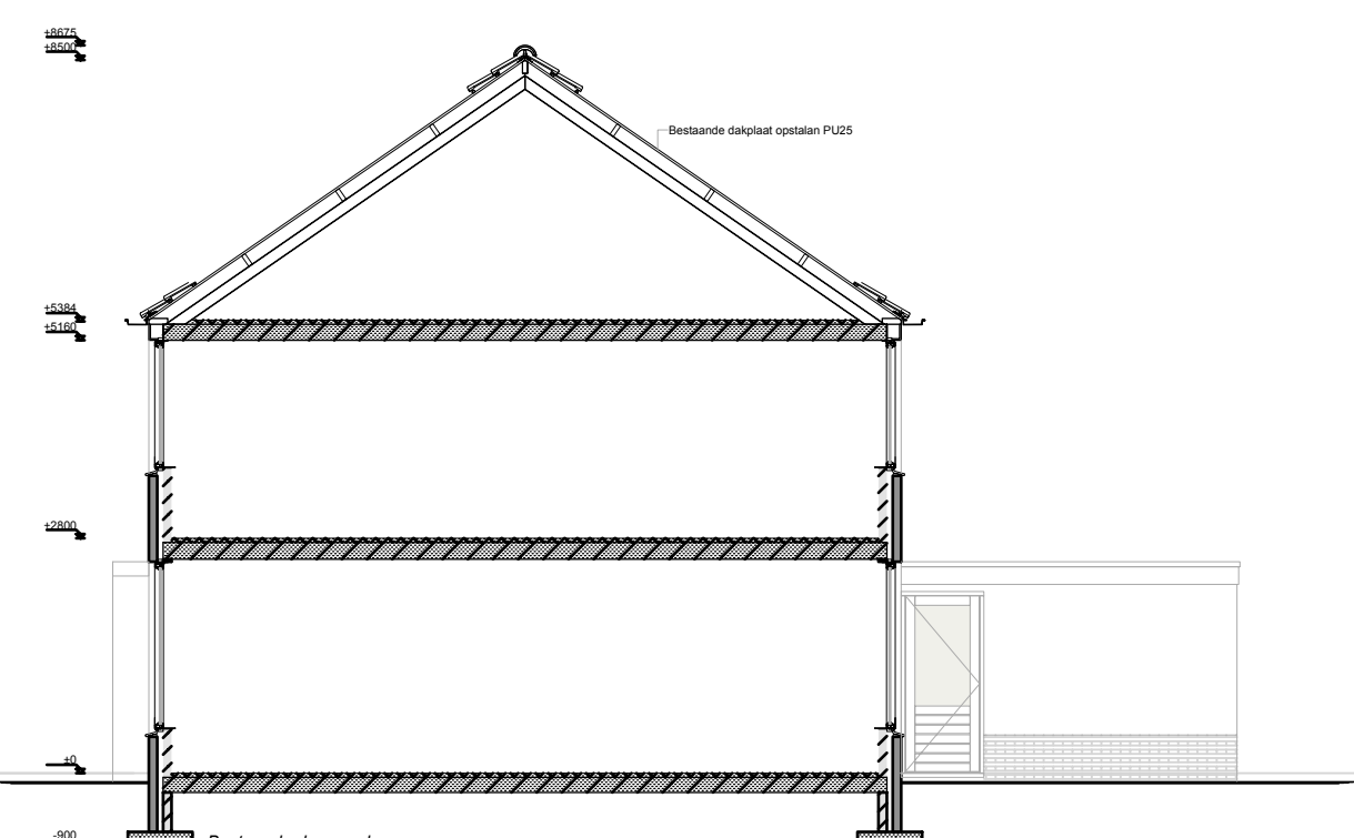
Bestaande deorside
