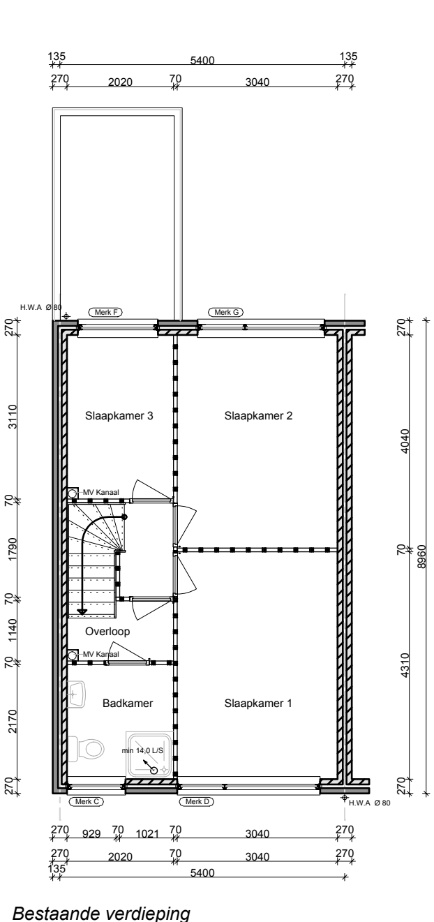
Bestaande verdieping
