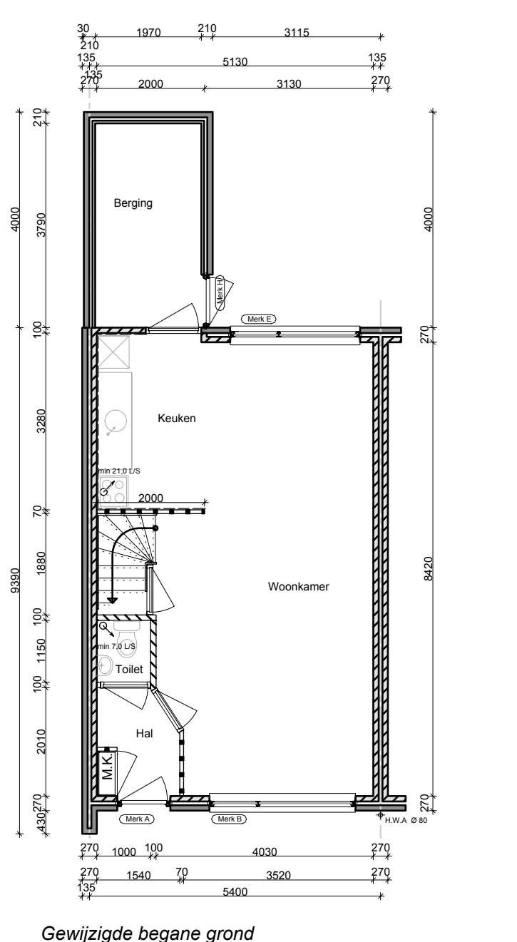
Gewijzigde begane grond
