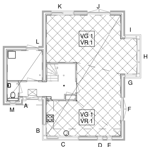
begane grond
