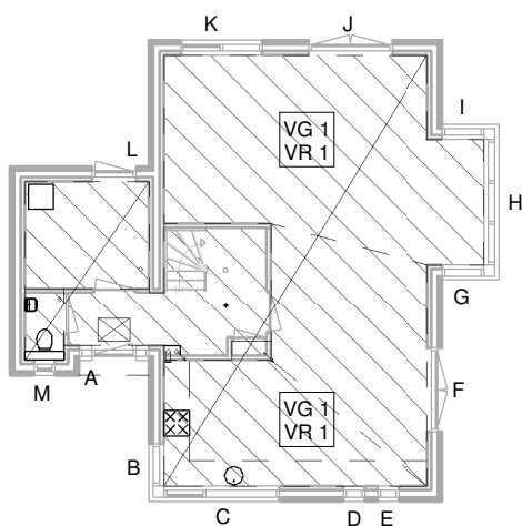
begane grond
