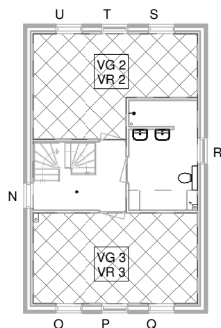
eerste verdieping
