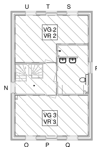
eerste verdieping
