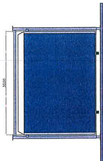
LINKERZIJTAANZICHT
