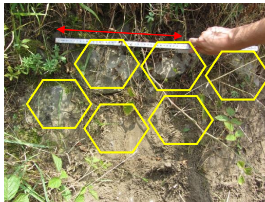
Figuur II-6 Zetsteen op driekwart van het talud bij 34,5 (rode pijl = 40 cm)
