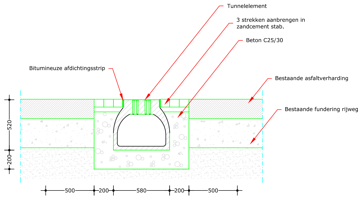
Principedoorsnede faunapassage (na aanleg)
