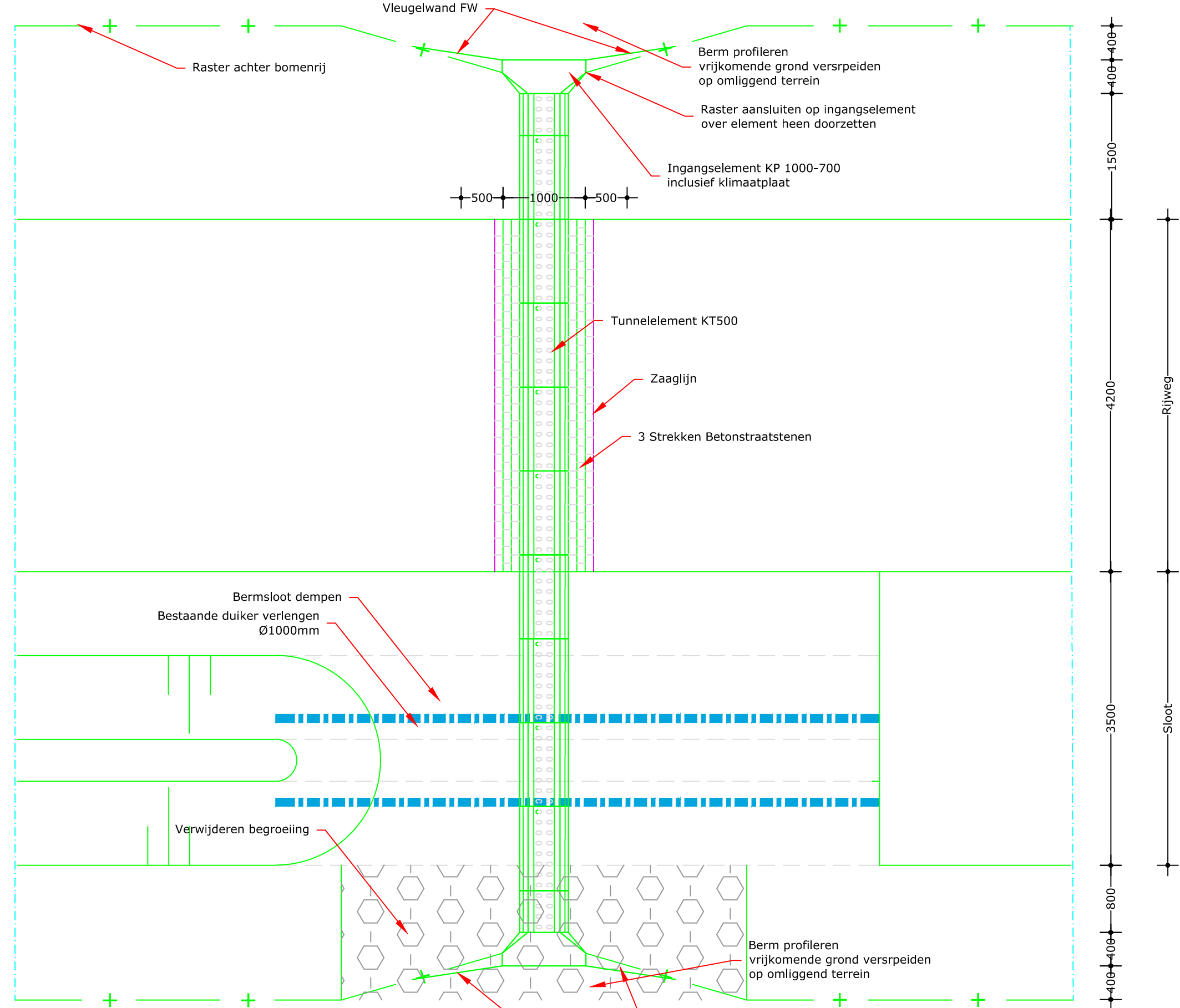
Detail faunapassage nabij Kasteel Elsloo locatie 1 (situatie na aanleg)
