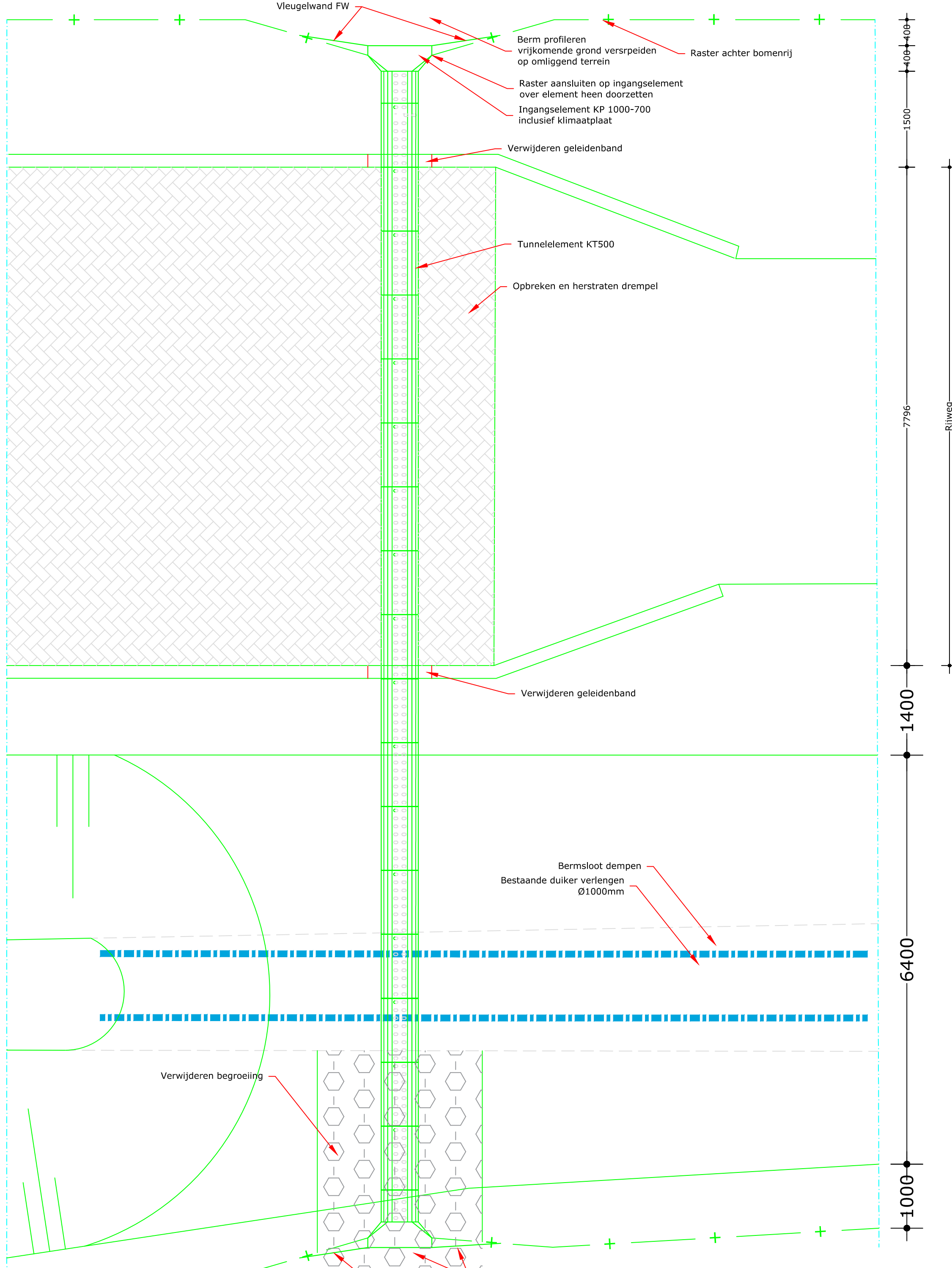
Detail faunapassage nabij Kasteel Elsloo locatie 2
