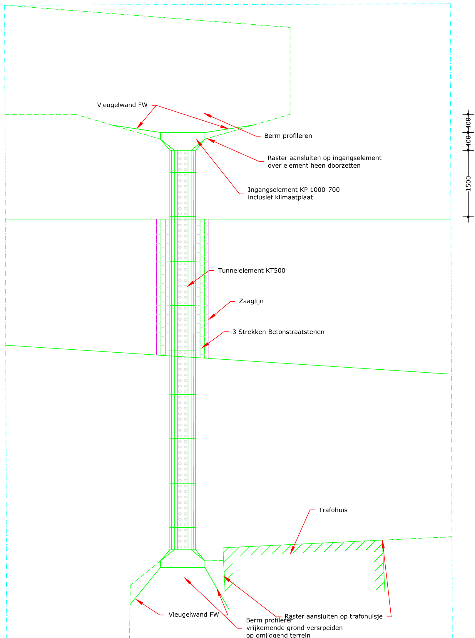
Detail faunapassage nabij Kasteel Elsloo locatie 3
