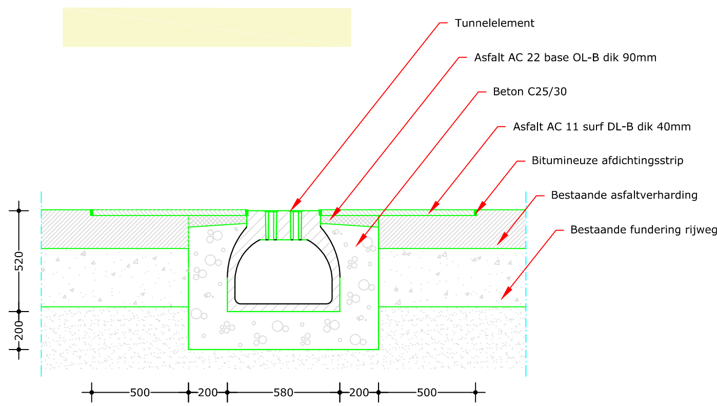
Principedoorsnede faunapassage (situatie na 1 jaar)
