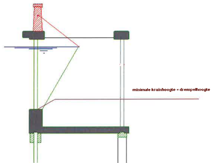
Zijaanzicht stuw
