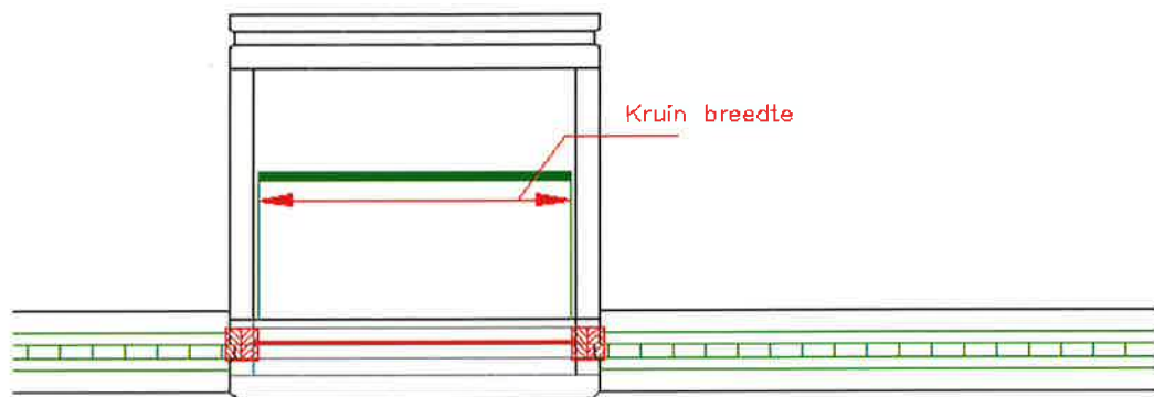
Bovenaanzicht stuw
