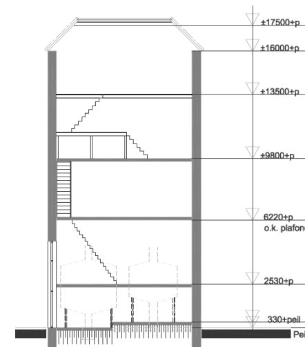
DOORSNEDE C-D:
