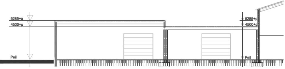
DOORSNEDE G-H:
