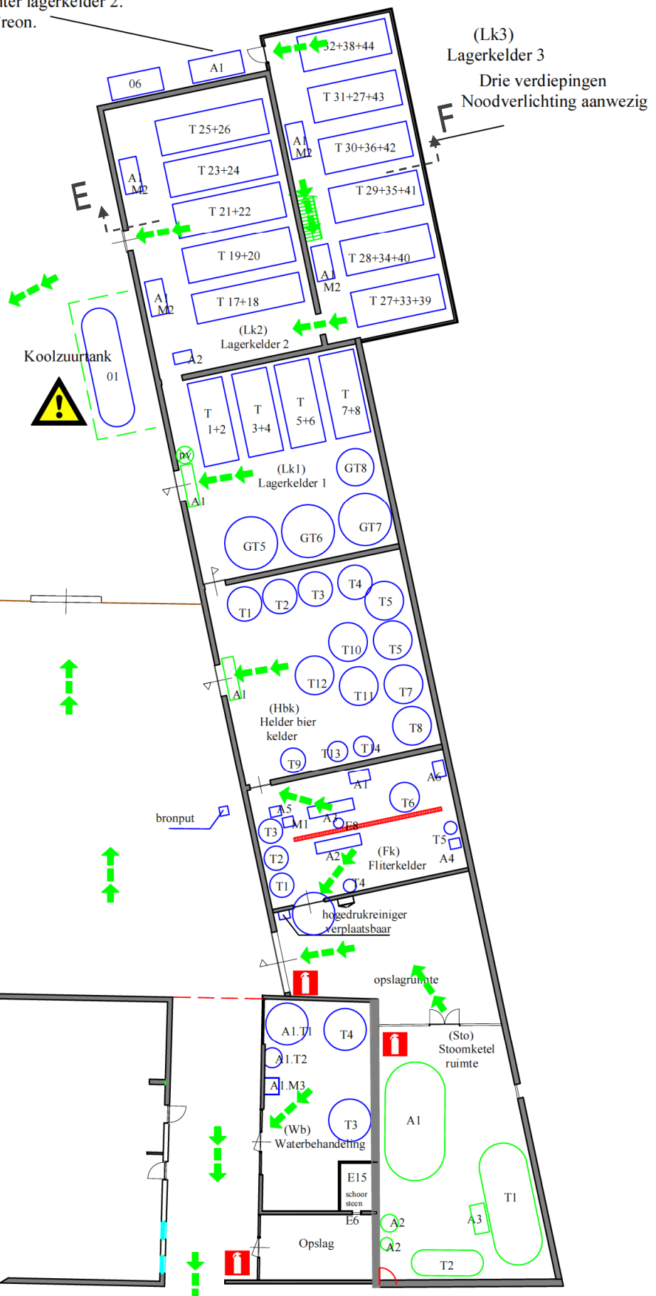
1° BOUWLAAG:
