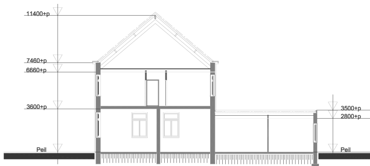
DOORSNEDE A-B:
