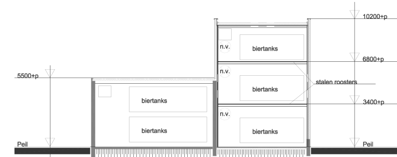
DOORSNEDE E-F:
