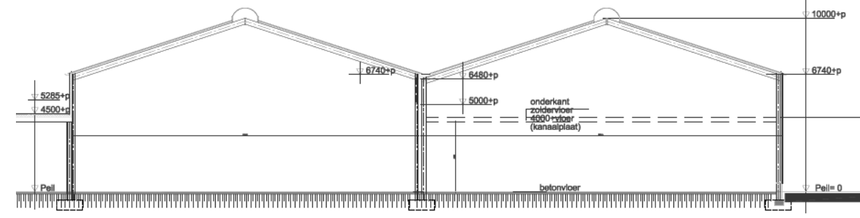
DOORSNEDE I-J:
