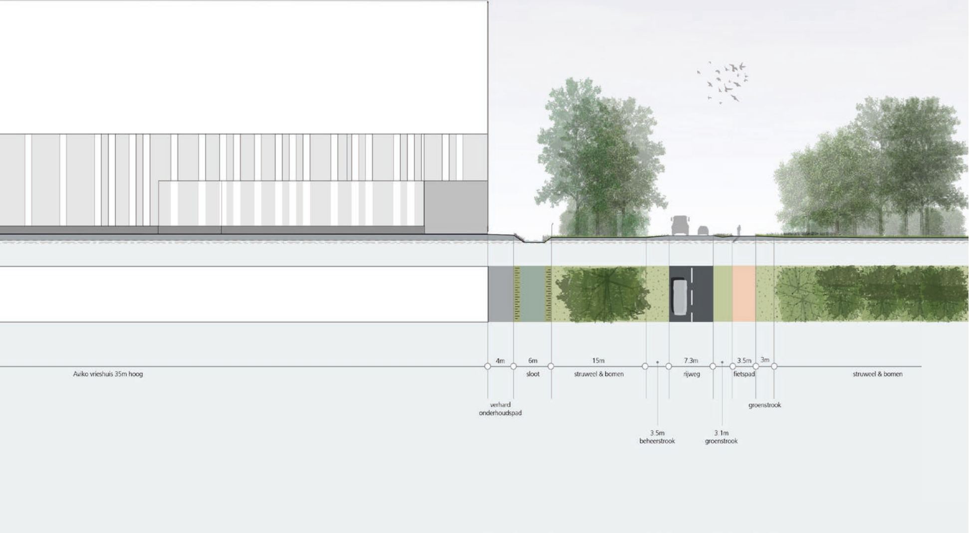
^ profiel overgang naar parkeerplaats
