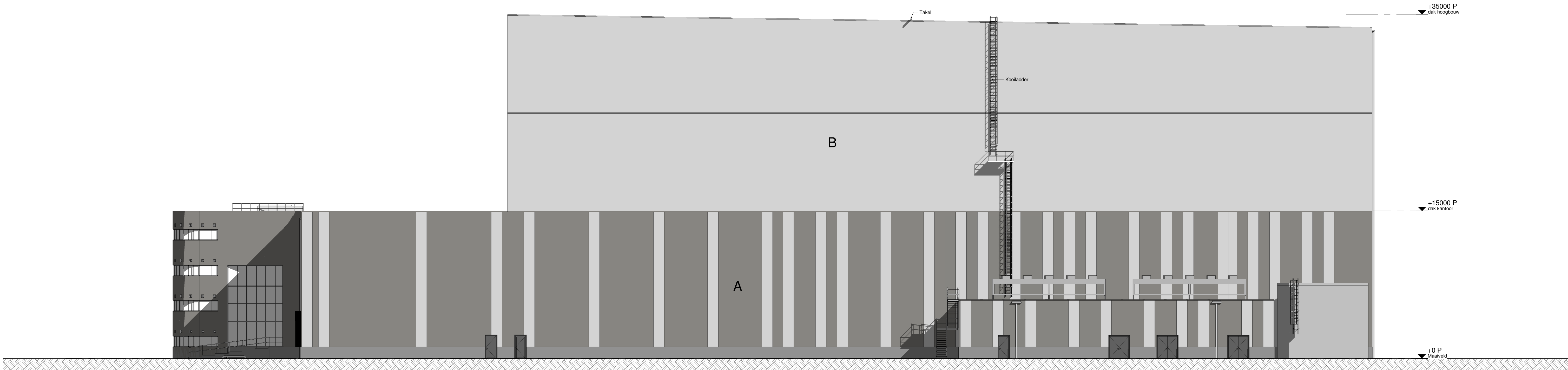
201 Zijgevel rechts 1 : 200
