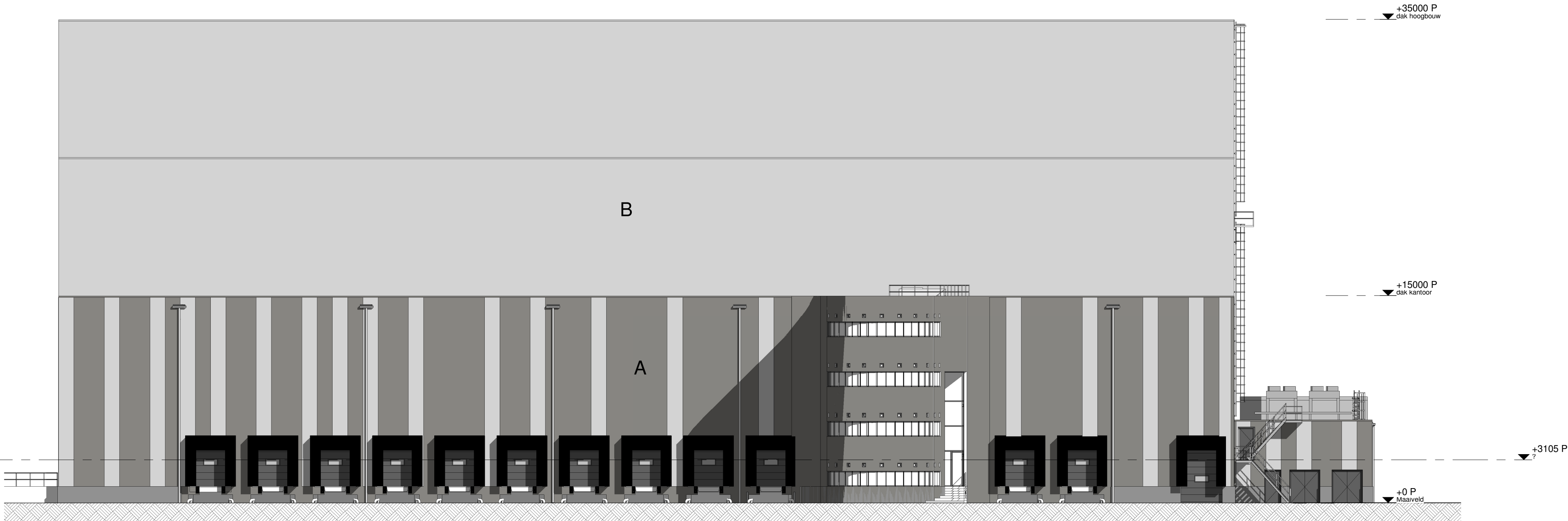
201 Voorgevel 1 : 200
