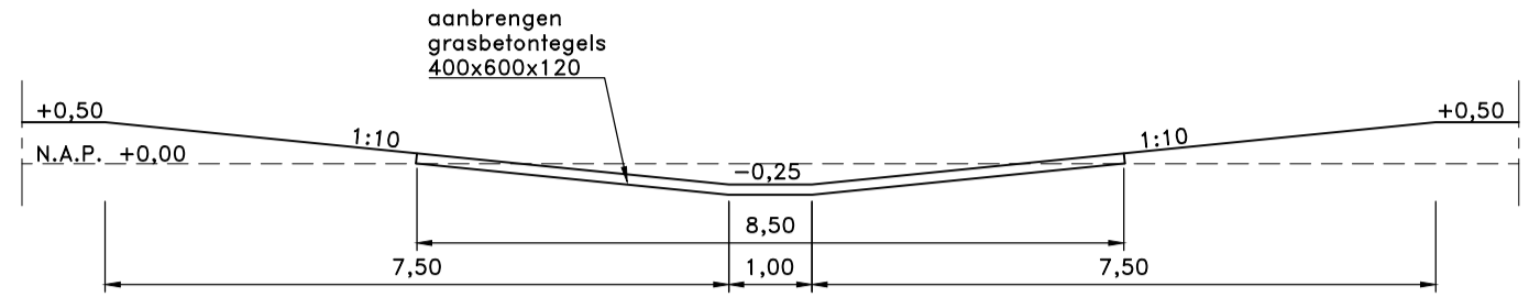
dwarsprofiel B-B schaal 1:100
