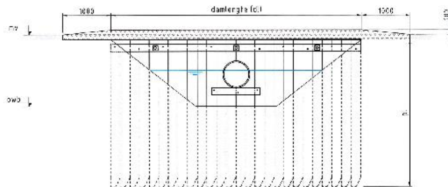
Voor aanzicht
