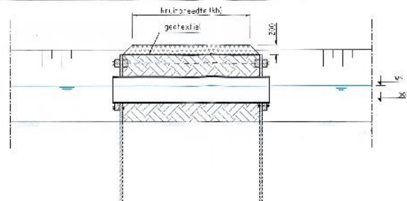
Doorsnede A-A'
