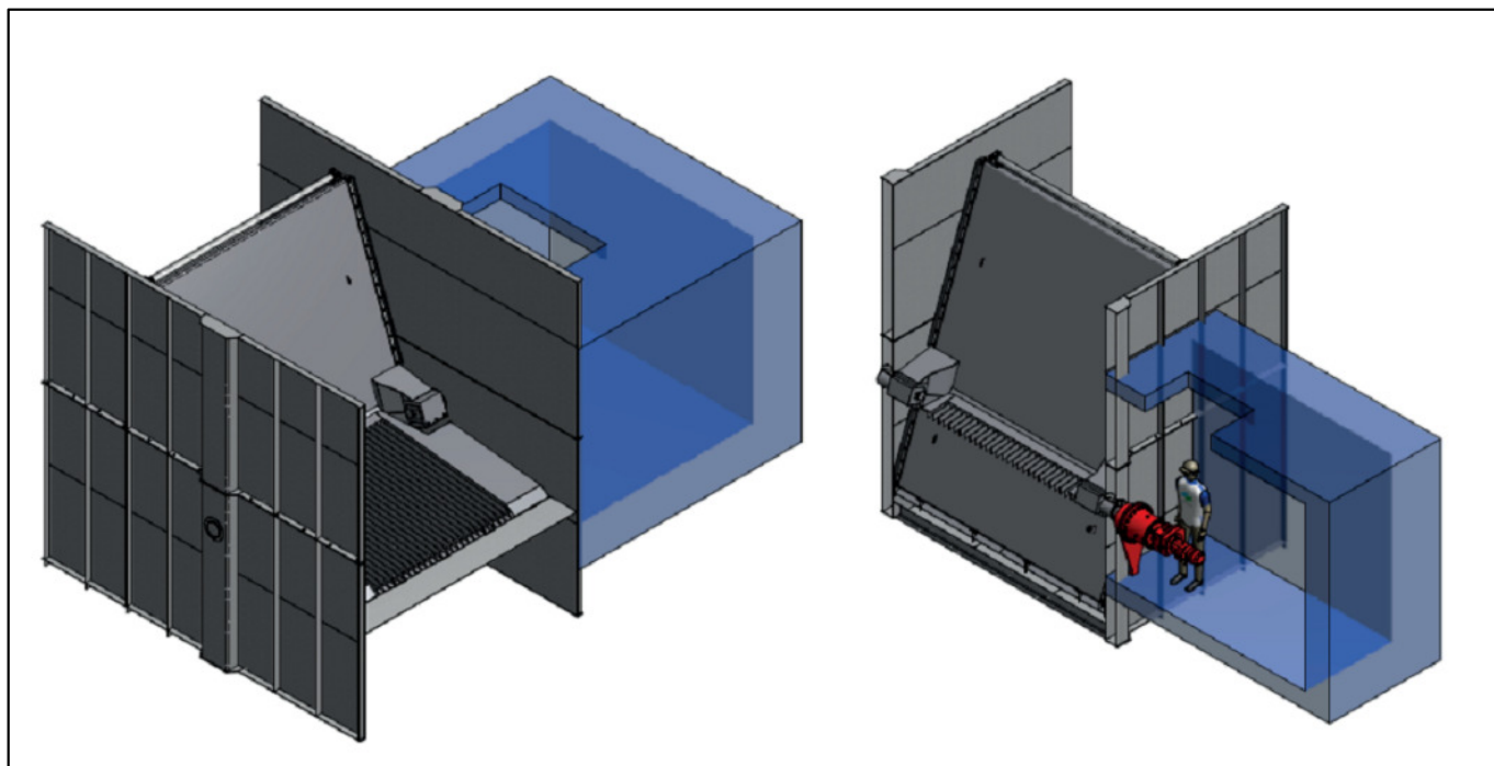
Figuur 17: vlinderklep in frame met de technische ruimte en aandrijving
