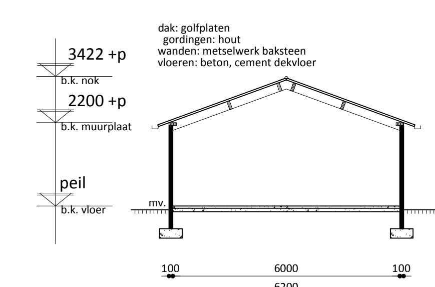
doorsnede D-D
