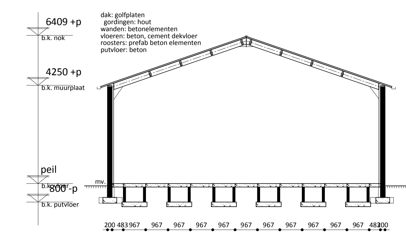
doorsnede C-C
