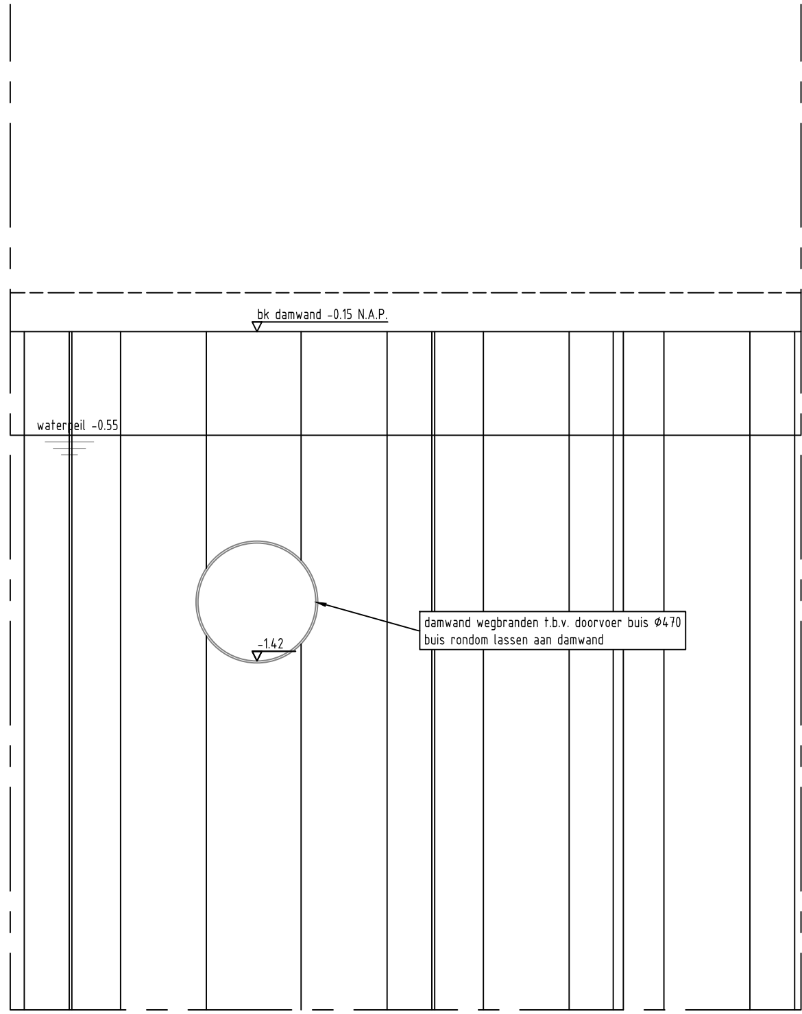
Vooraanzicht Schaal 1:50
