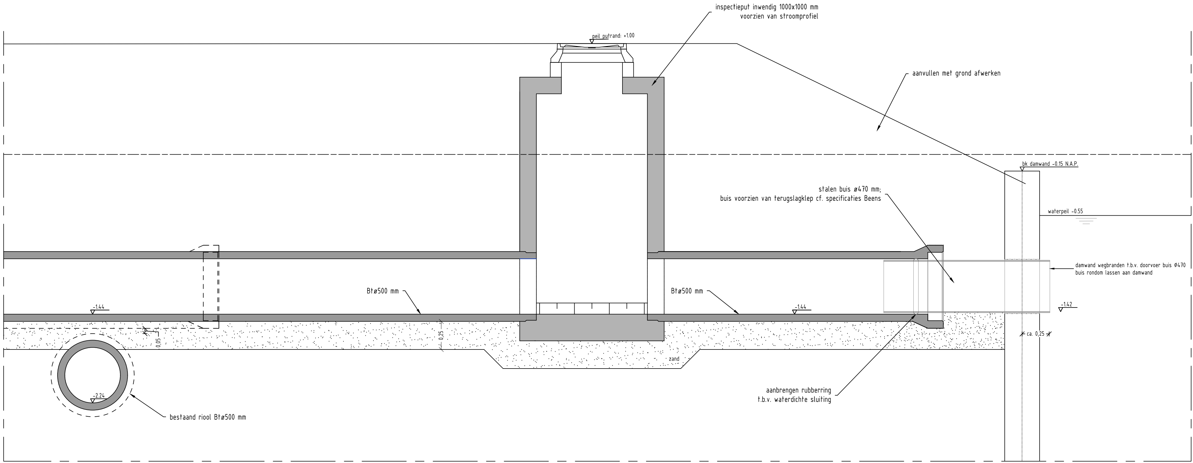
Dwarsprofiel 1 Schaal 1:50
