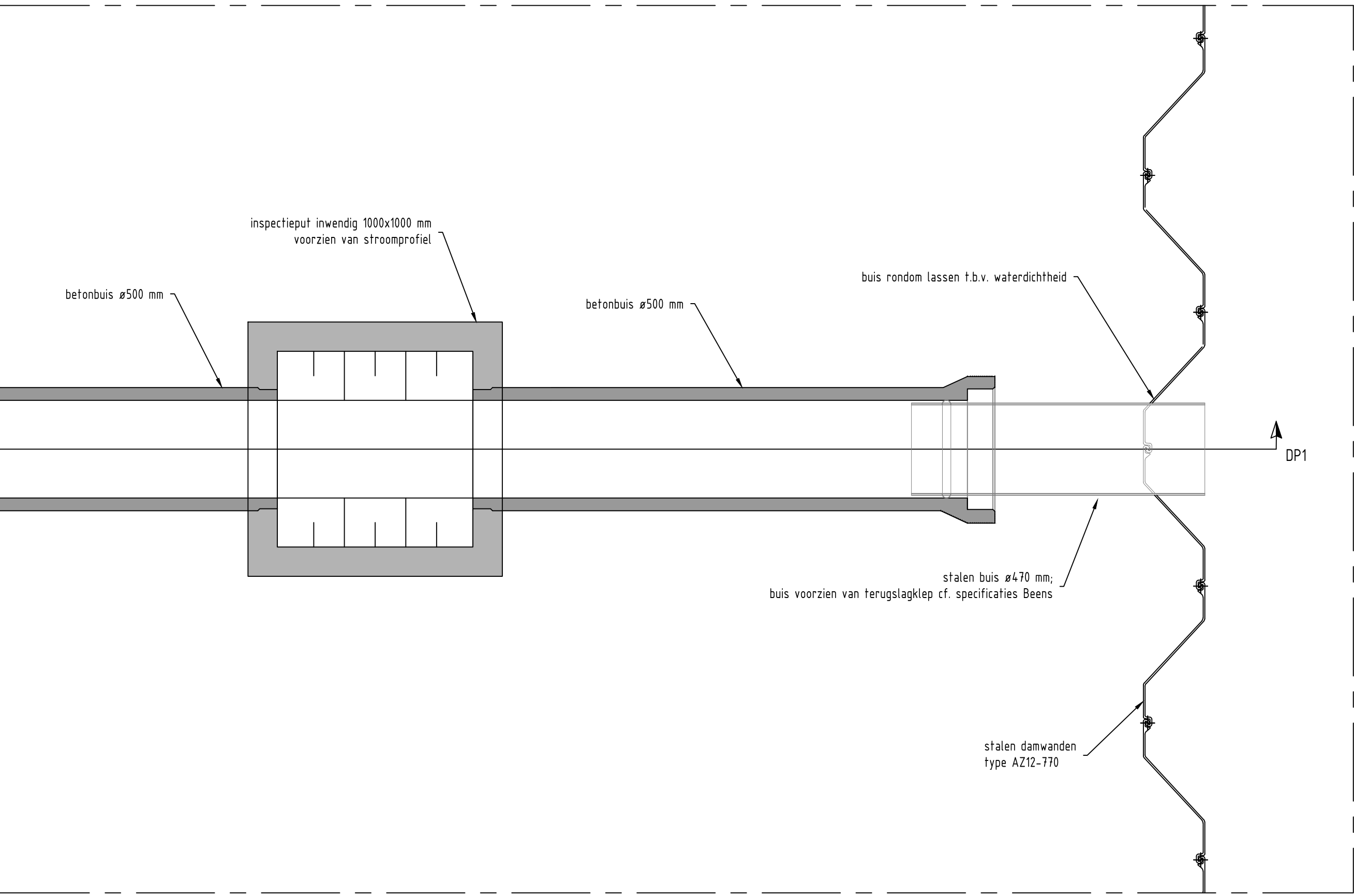
Bovenaanzicht Schaal 1:50
