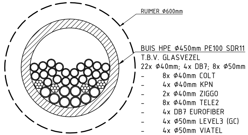
DOORSNEDE BORING SCHAAL 1:10
