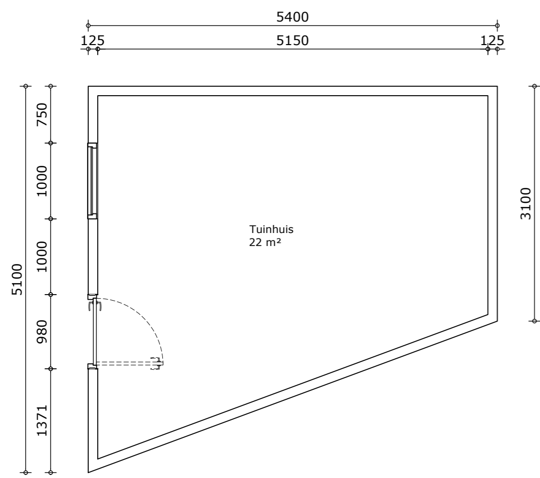
Beganegrond
