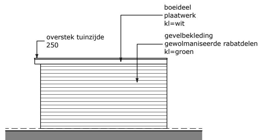
Voorgevel
