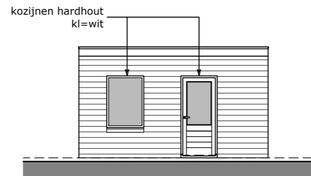
L zijgevel
