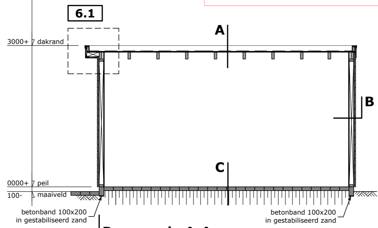
Doorsnede A-A
