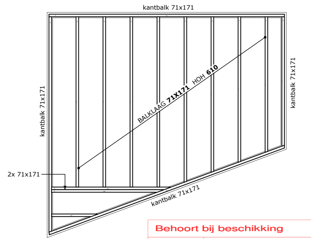
Balklagen
