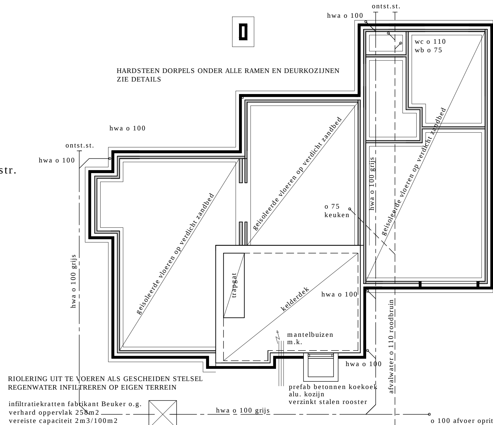
KELDERDEK - FUNDERING - RIOLERING BEGANE GRONDVLOER
