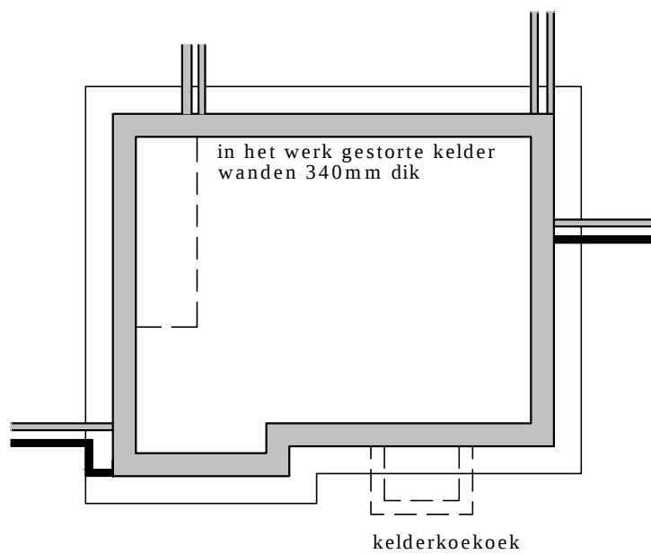
KELDERVLOER EN WANDEN
