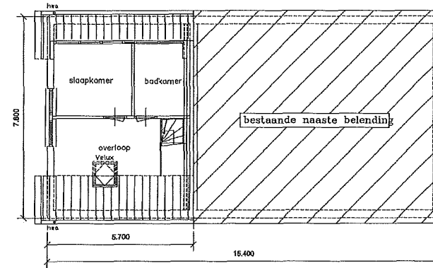
bestaande verdieping
