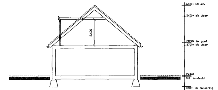
bestaande doorsnede
