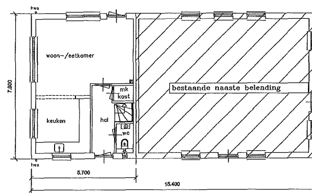
bestaande begane grond ok plafond ≈ 2470mm
