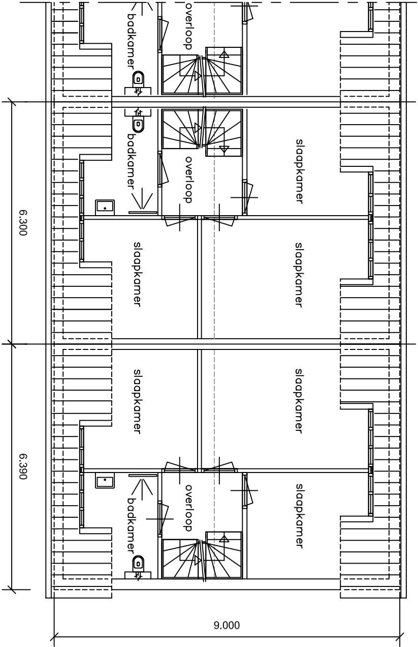
bestaande verdieping
