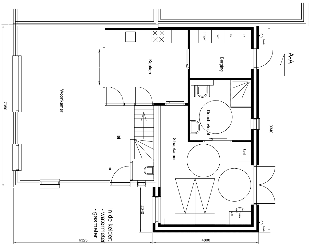
Begane grond nieuw
