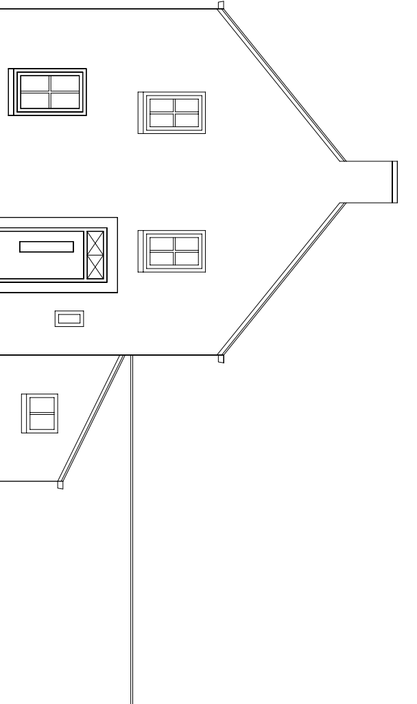
Rechter zijgevel bestaand
