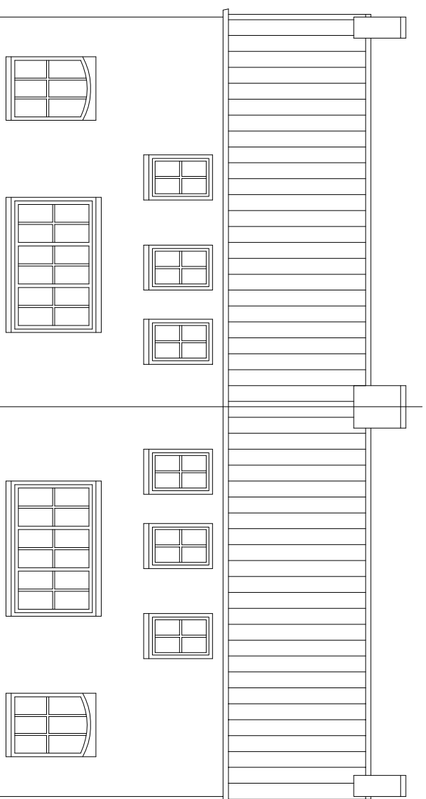
Voorgevel bestand
