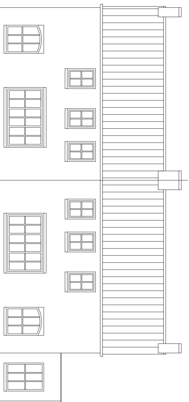
Voorgevel Nieuw
