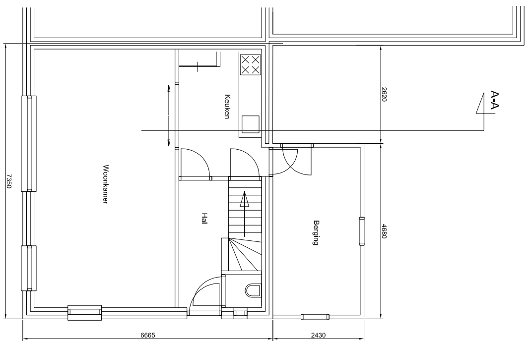
Begane grond bestand
