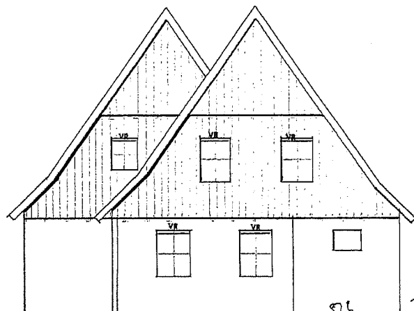
ACHTERGEVEL
