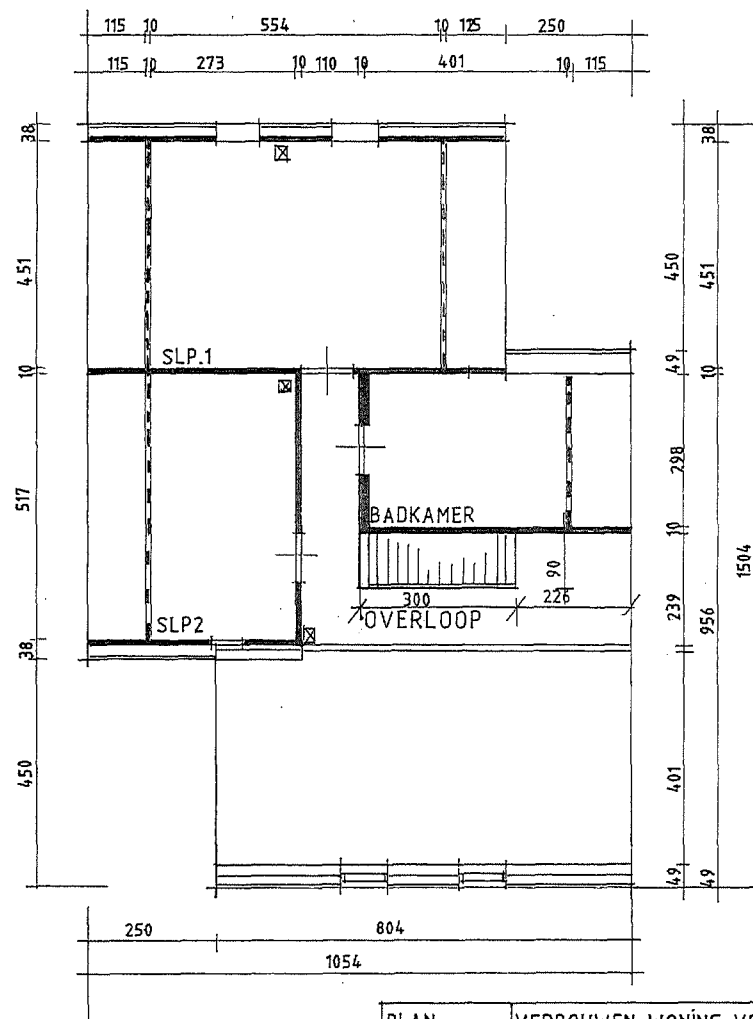
VERDIEPING
