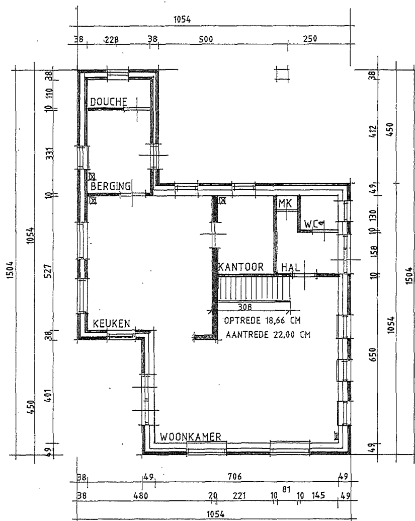
BEGANEGROND
