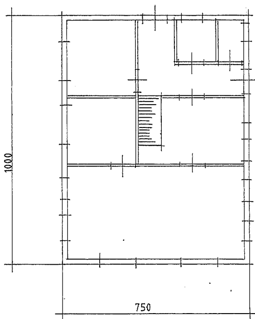
BEGANEGROND
