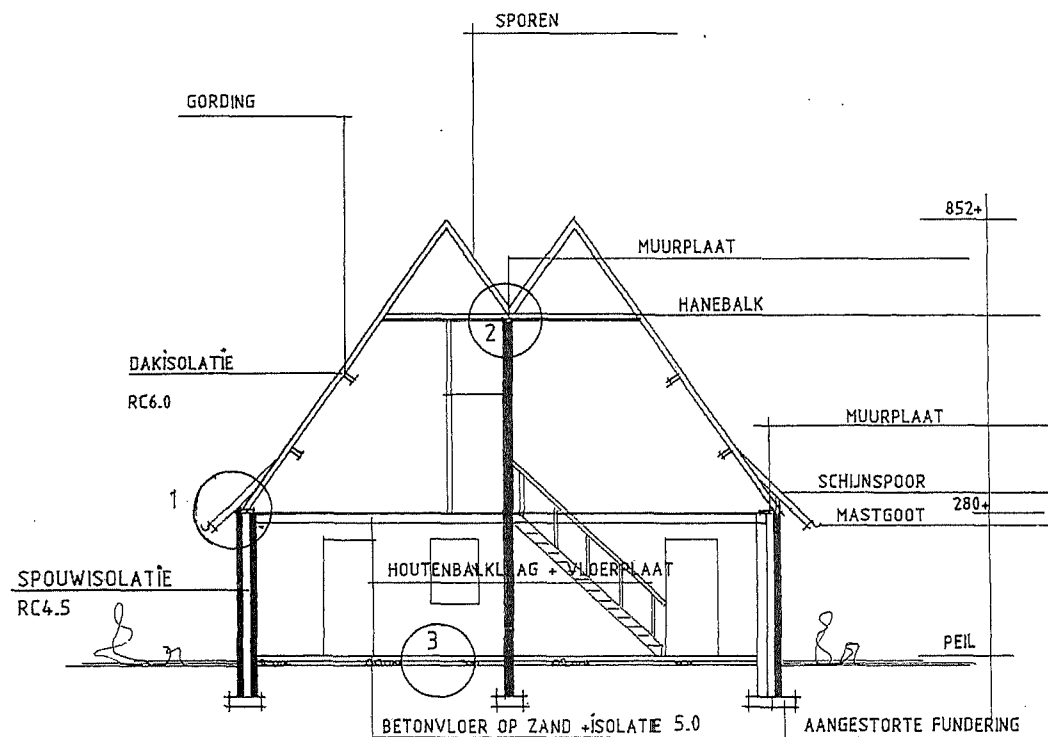
DOORSNEDE A-A
