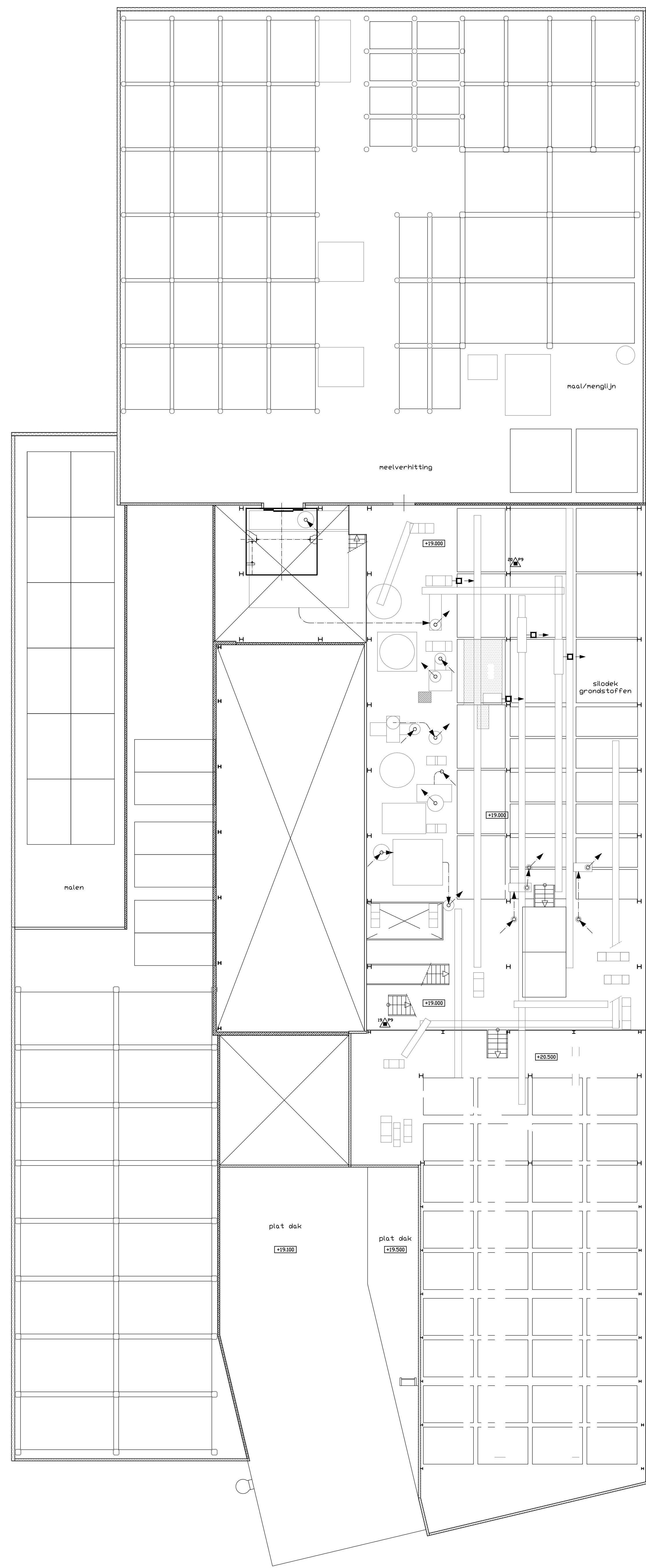
vloeren / daken 19 meter
