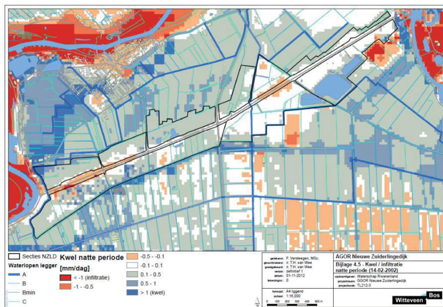
Afbeelding II.4. Kwel in natte periode
