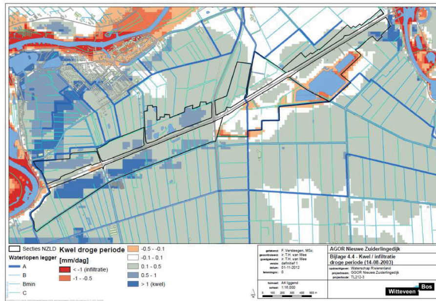
Afbeelding II.5. Kwel in droge periode
