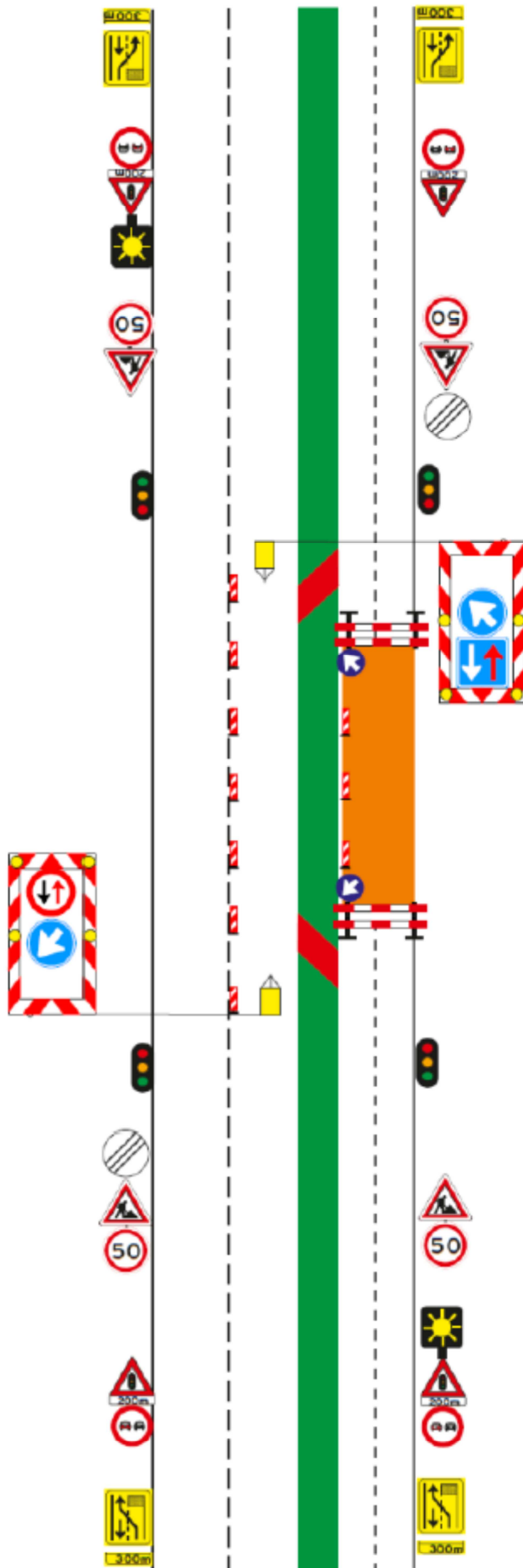
Figuur 5, CROW 1306C + 1124B
