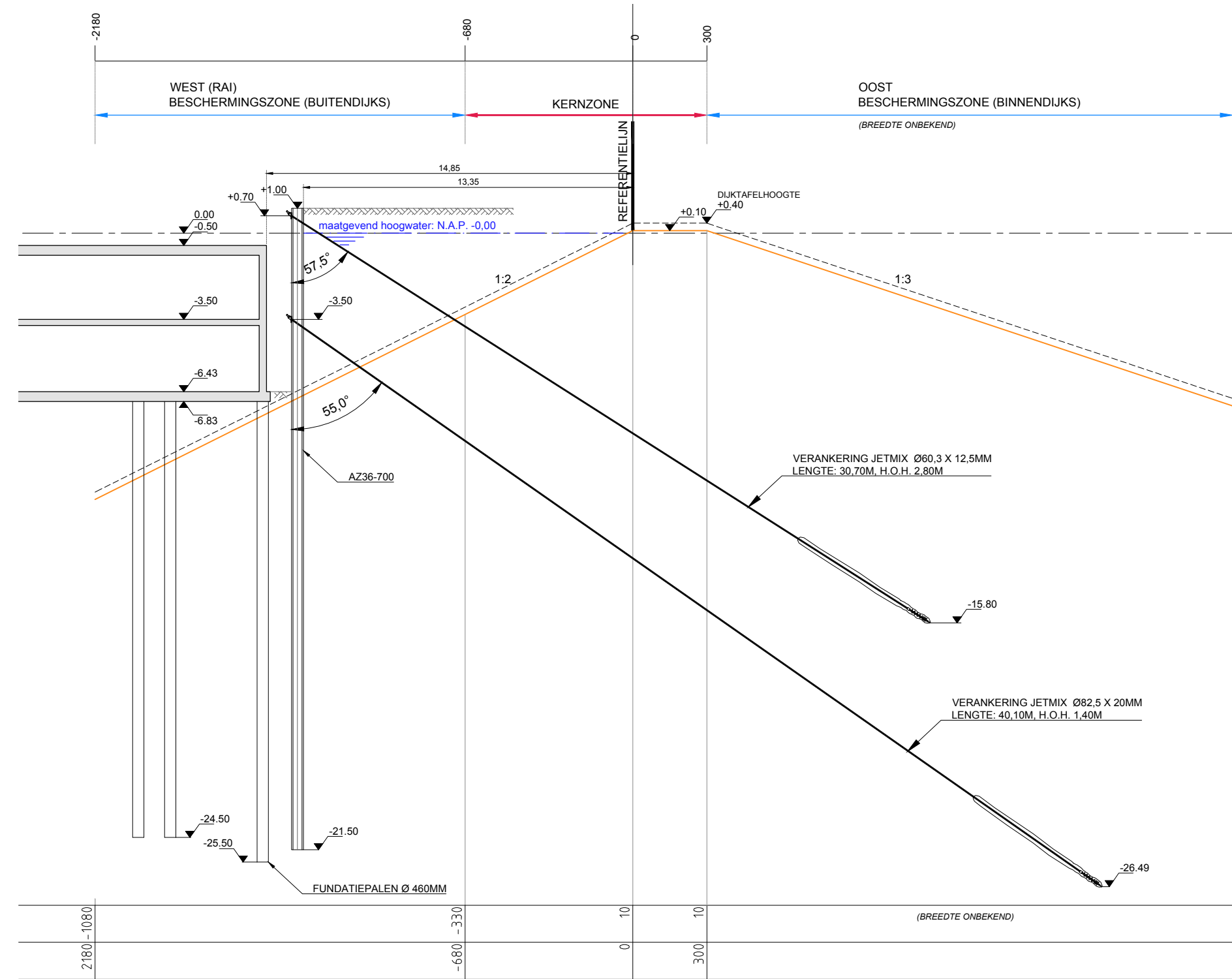
DOORSNEDE A-A 1:200
