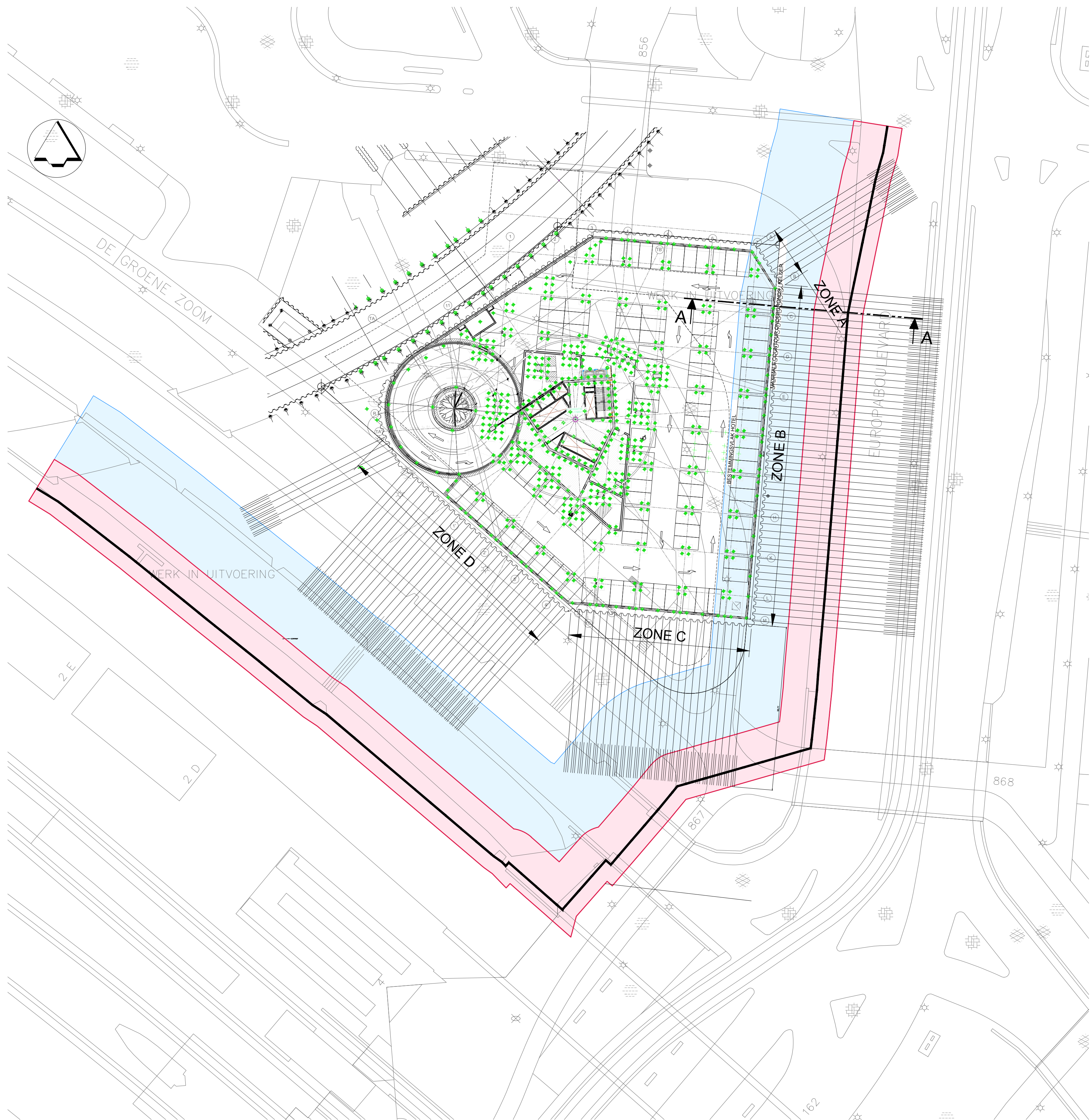
PLANOVERZICHT 1:500
