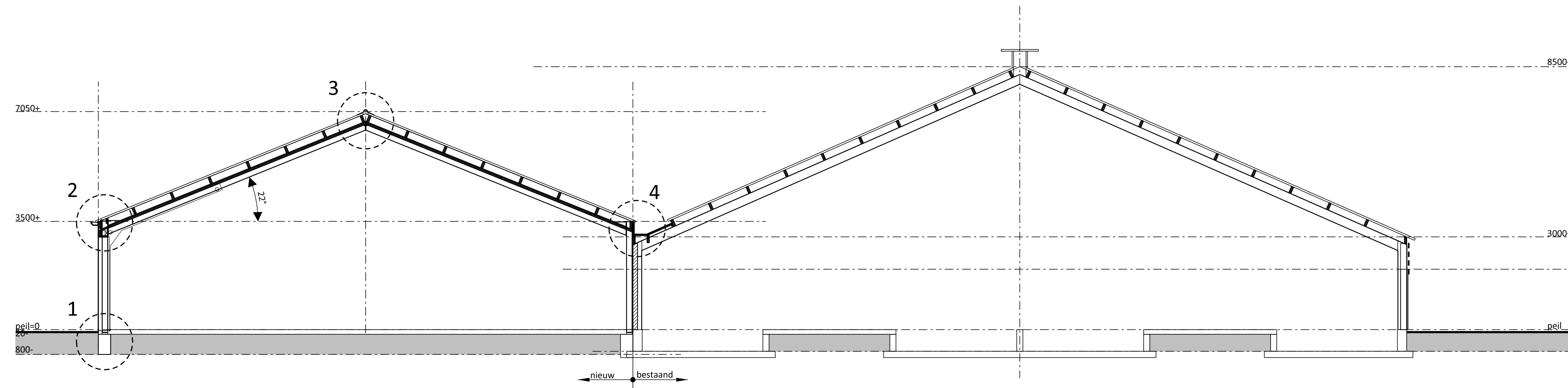
Doorsnede A-A
