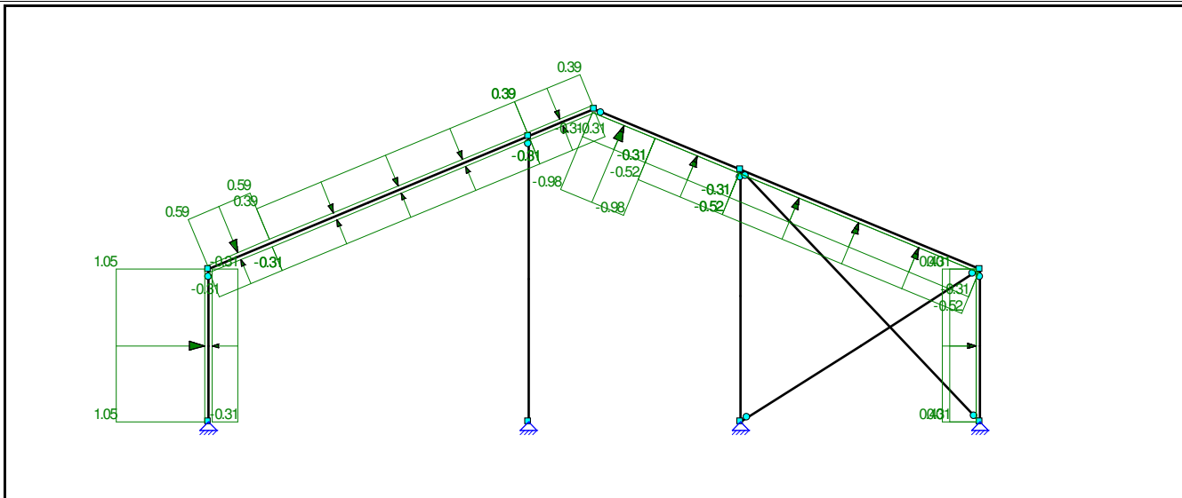
B.G.5: WINDBELASTING VAN LINKS + OVERDRUK (ZADELDAK FGH 2E CPE + IJ 1E CPE)
