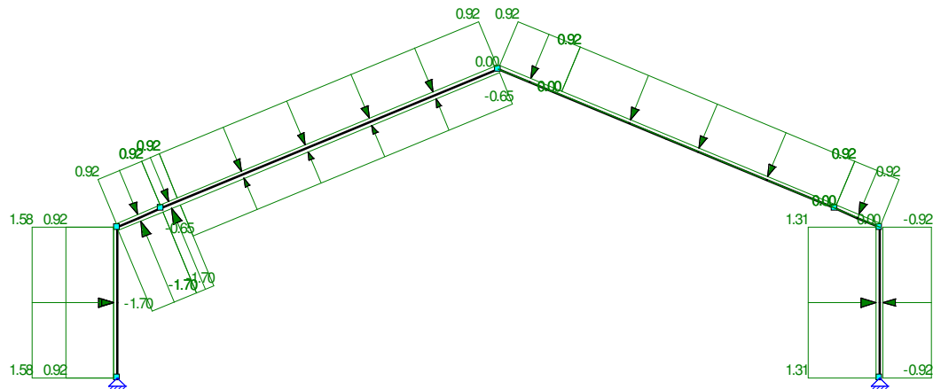
B.G.16: WINDBELASTING VAN LINKS + ONDERDRUK (ZADELDAK FGH 1E CPE + IJ 2E CPE) (2E CORR. FACTOR)
