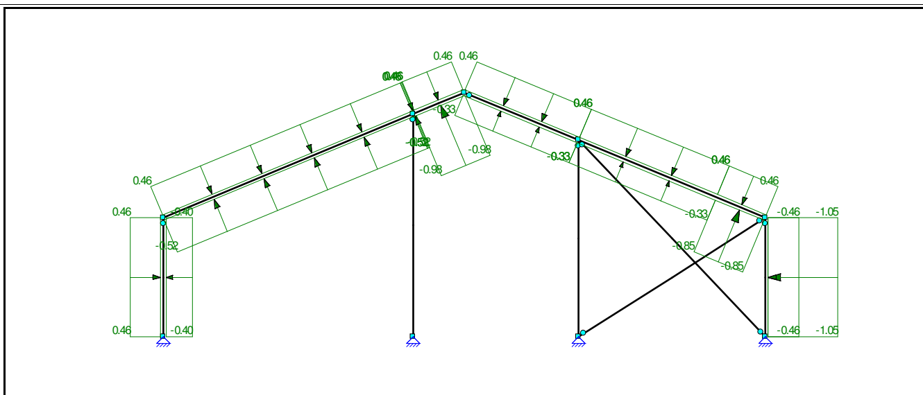
B.G.26: WINDBELASTING VAN RECHTS + ONDERDRUK
