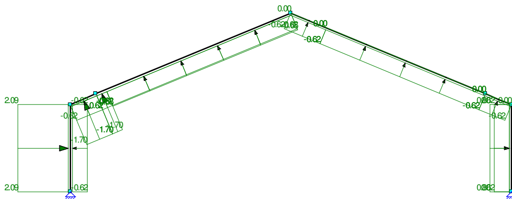
B.G.4: WINDBELASTING VAN LINKS + OVERDRUK (ZADELDAK FGH 1E CPE + IJ 2E CPE)
