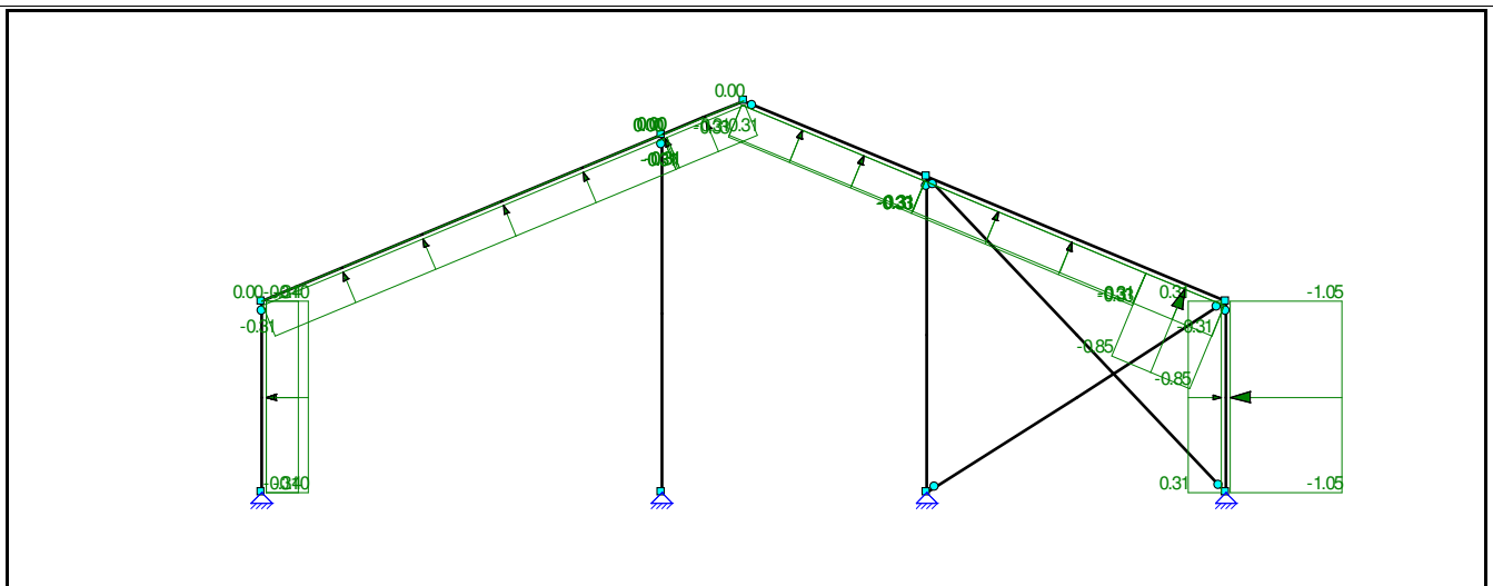
B.G.20: WINDBELASTING VAN RECHTS + OVERDRUK (ZADELDAK FGH 1E CPE + IJ 2E CPE)
