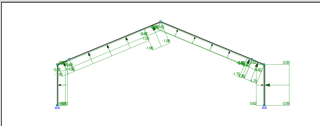
B.G.18: WINDBELASTING VAN RECHTS + OVERDRUK
