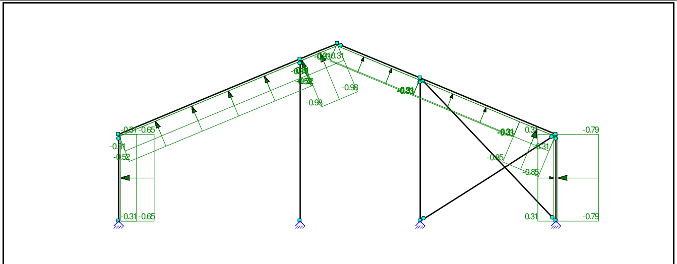
B.G.22: WINDBELASTING VAN RECHTS + OVERDRUK (2E CORR. FACTOR)
