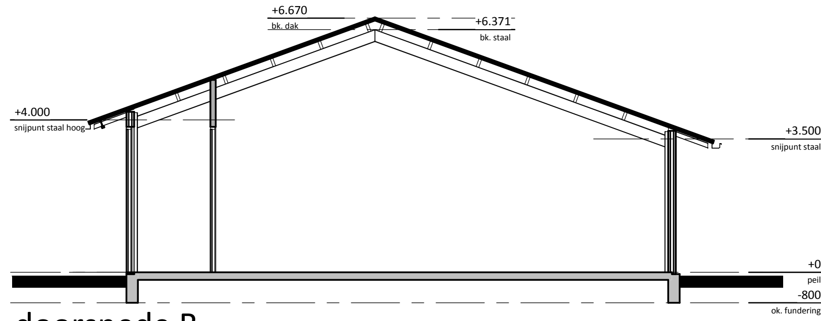
doorsnede B
