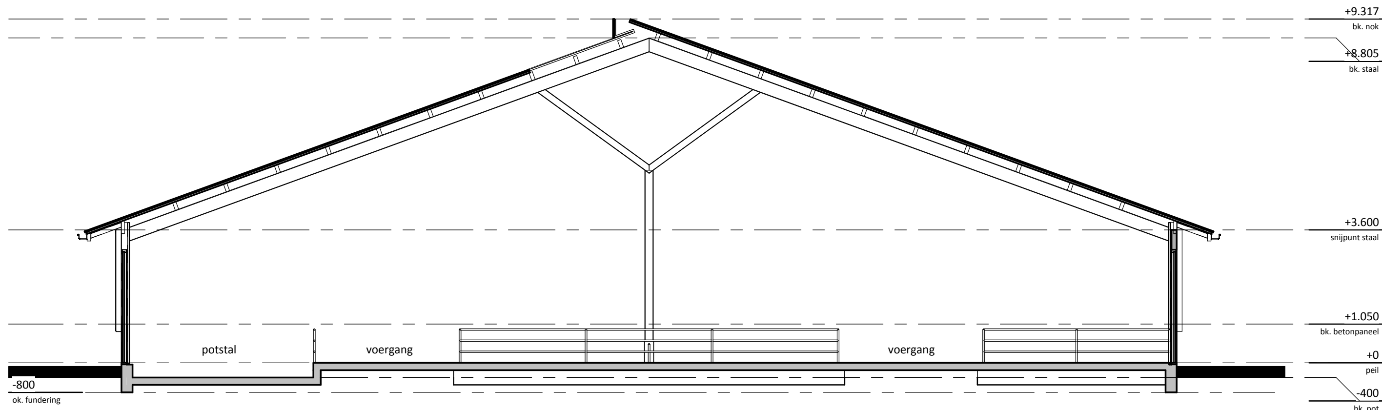
doorsnede C
