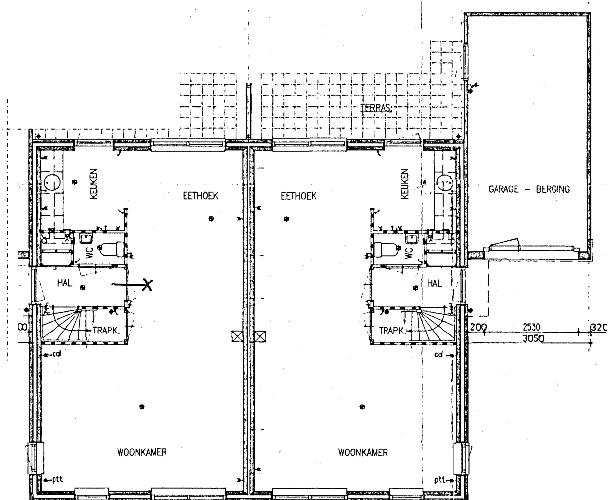
PLATTEGROND BESTAAND
