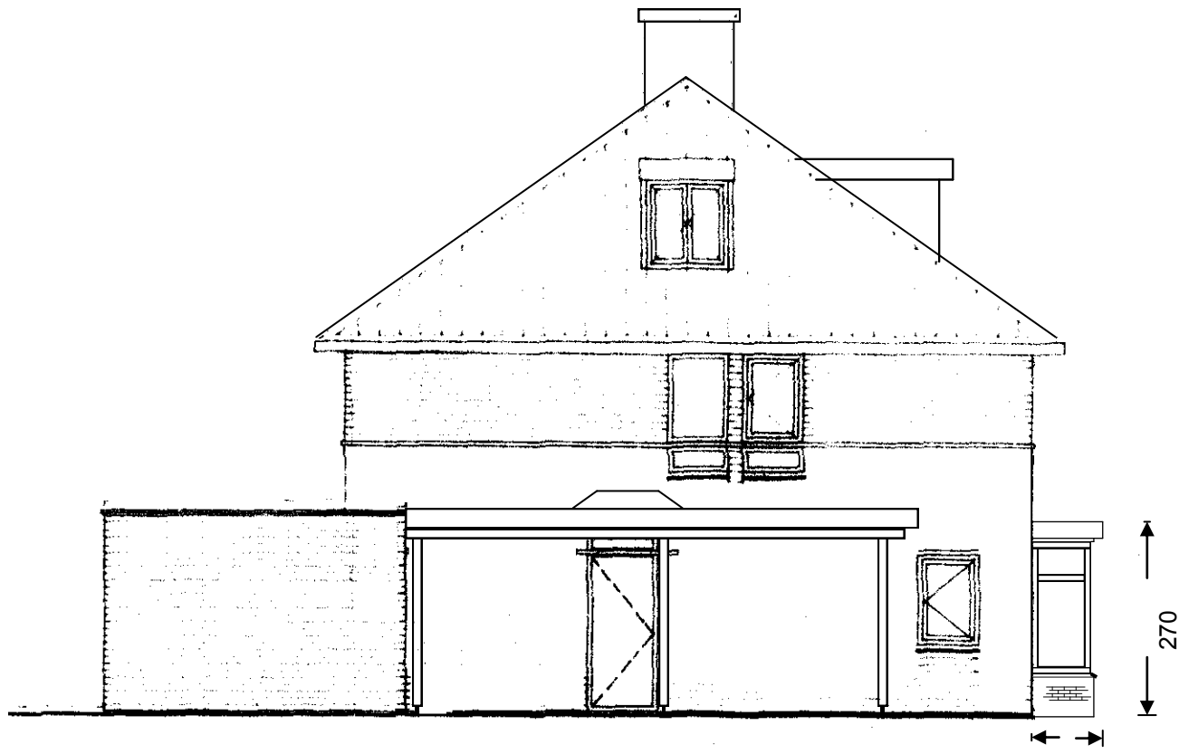
ZIJGEVEL NIEUW
