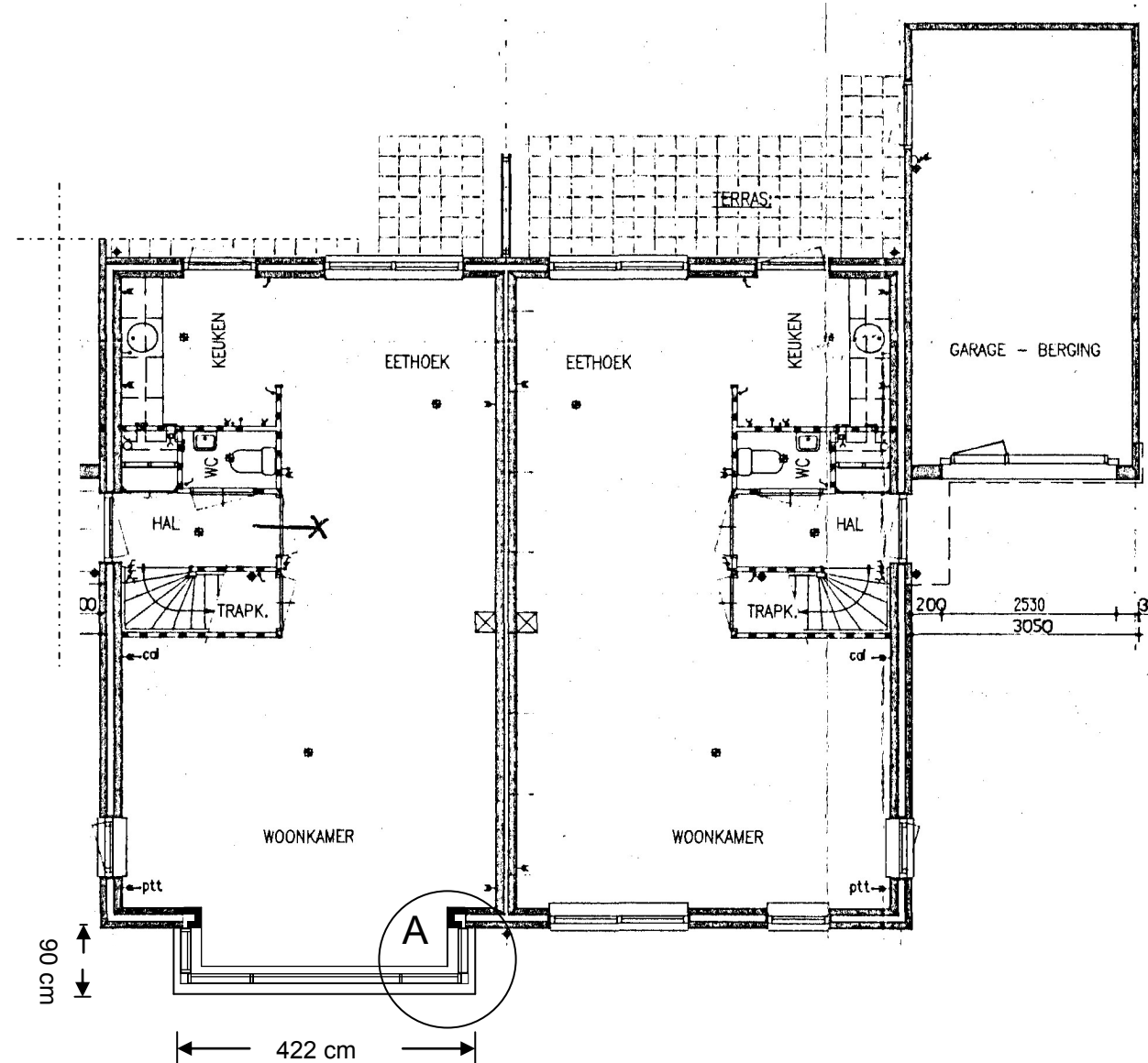
PLATTEGROND NIEUW
