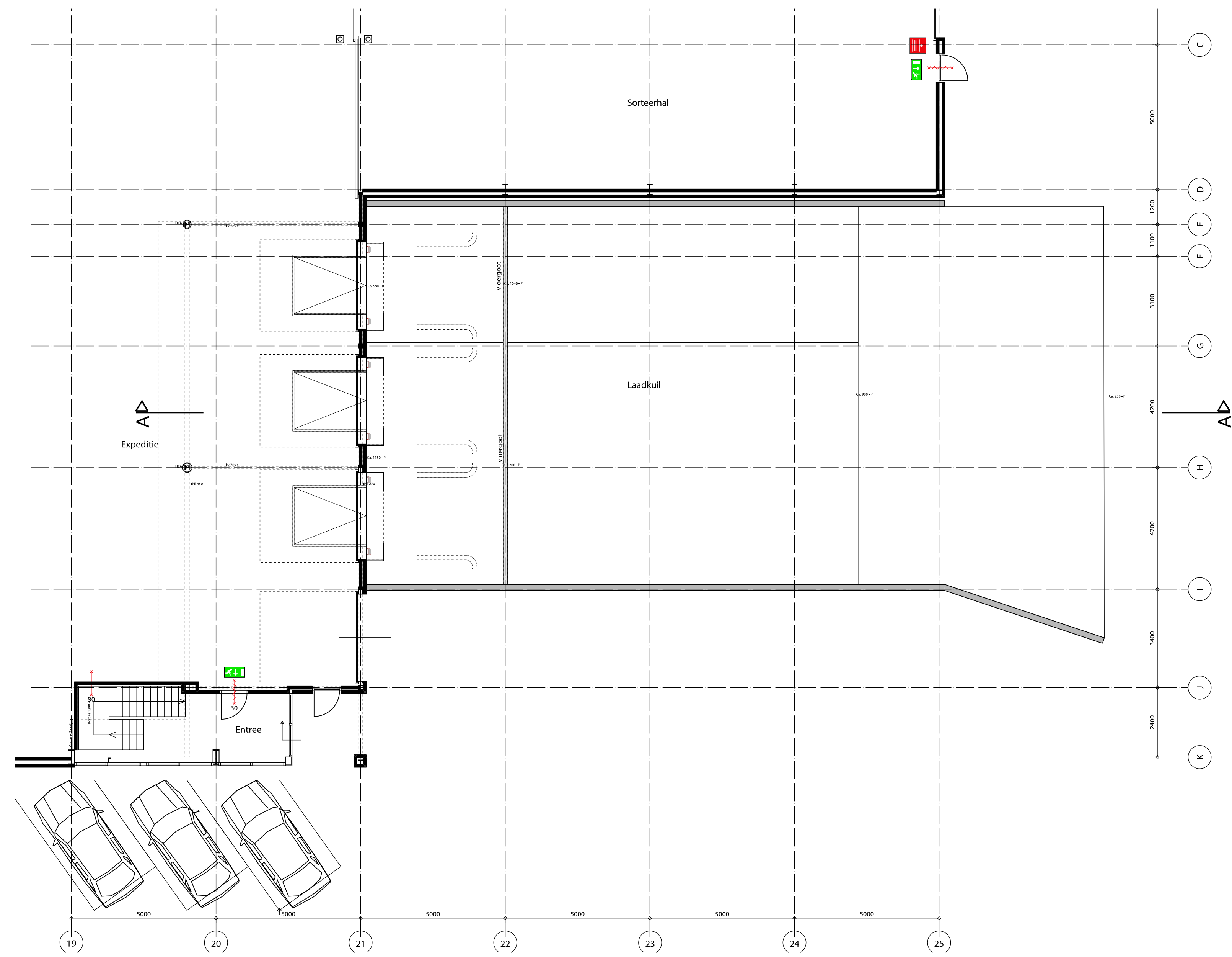
Begane grond
